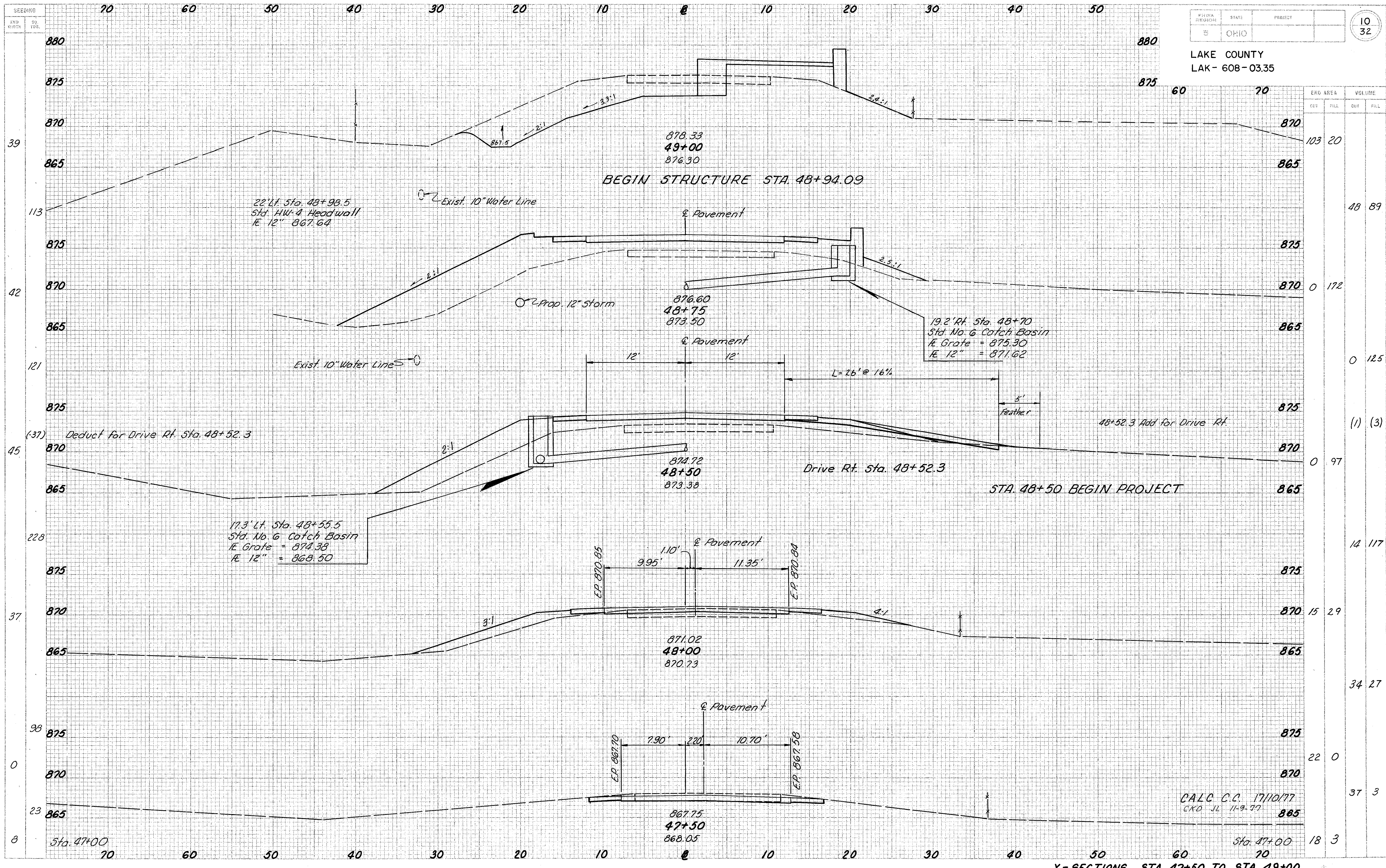
X-SECTIONS STA. 47+50 TO STA. 49+00
