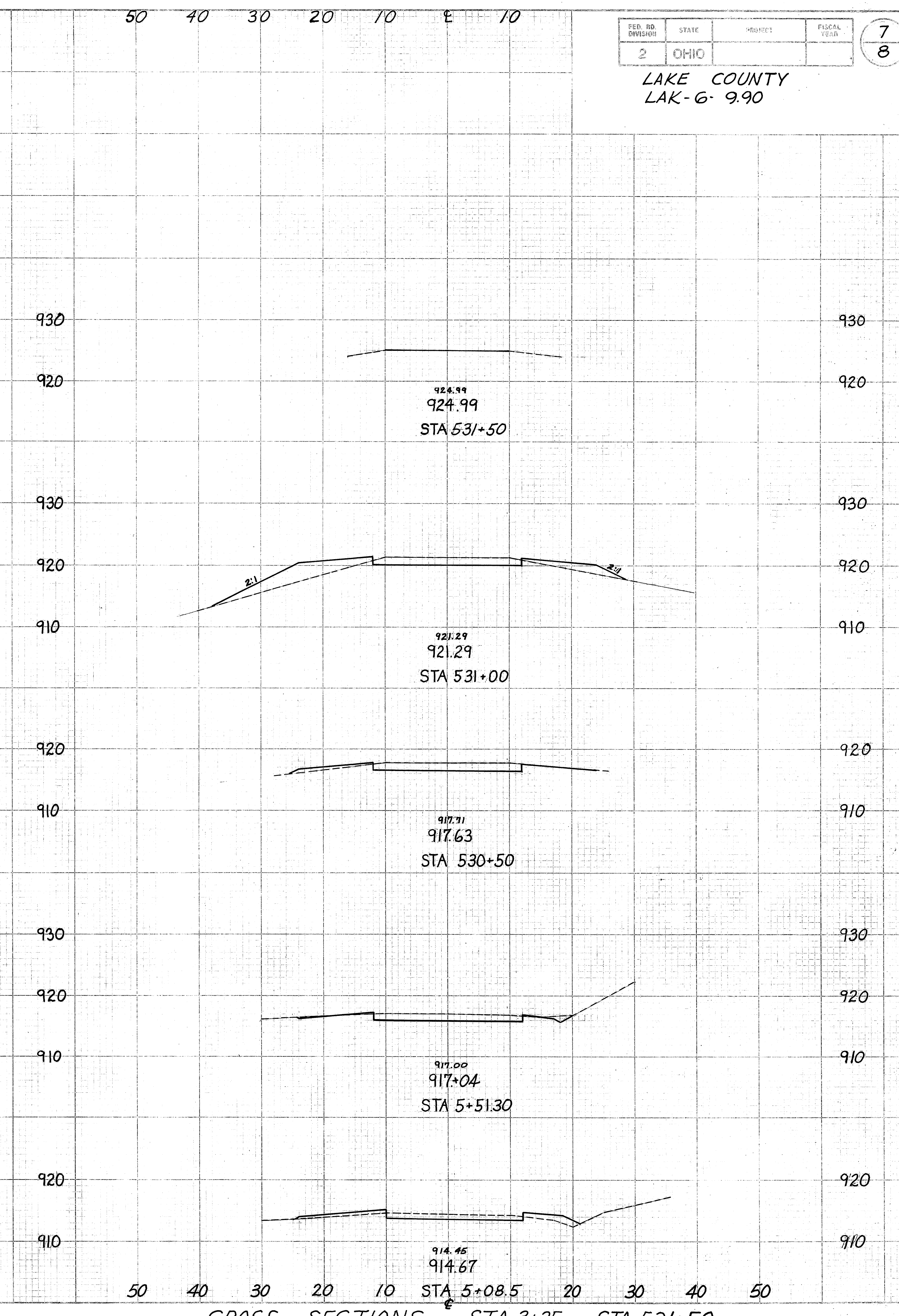
CROSS SECTIONS STA 3+35 TO STA. 531+50
