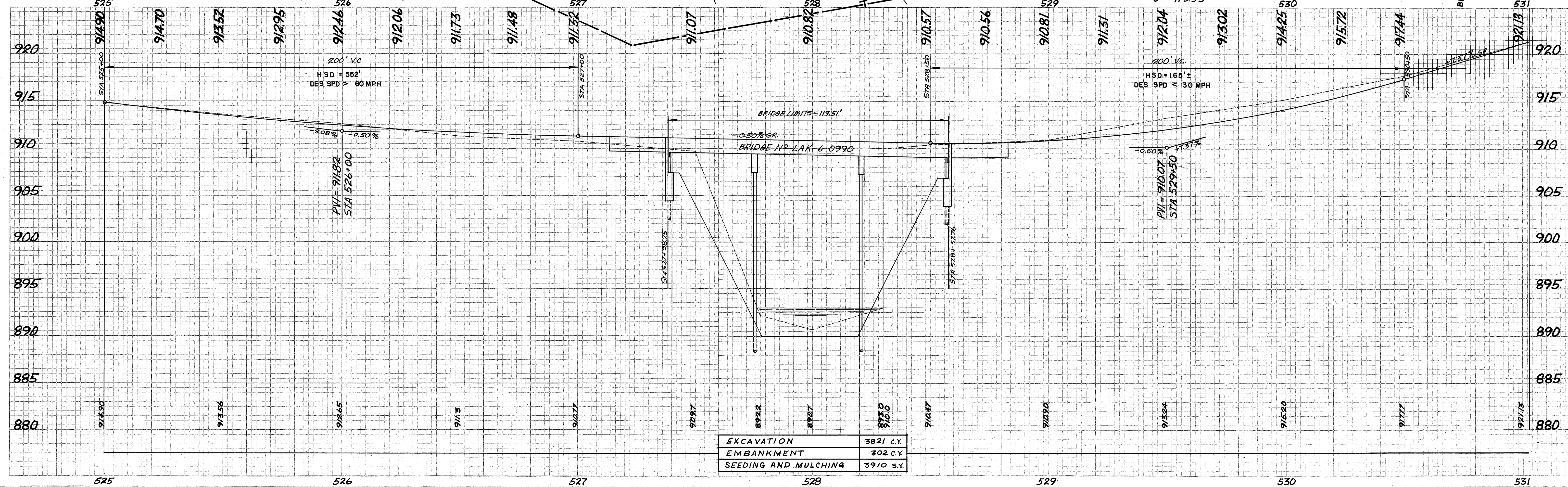
PLAN & PROFILE STA 525+00 TO PRC STA 531+02.43 (BACK)
