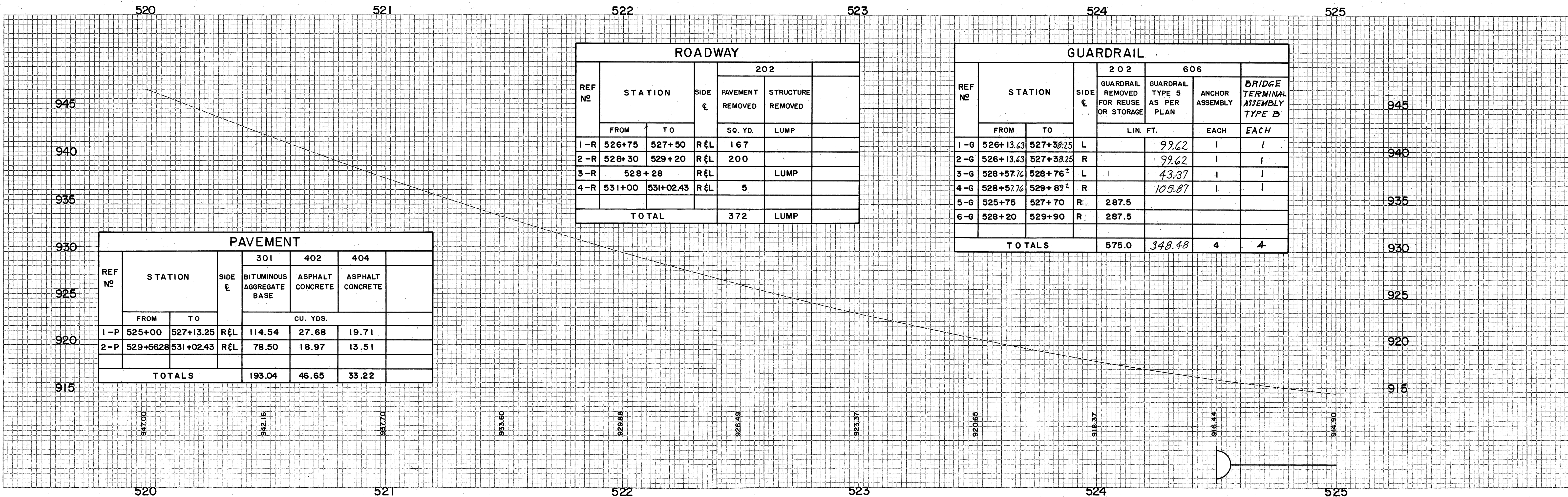
PLAN & PROFILE... STA. 520+00 TO STA. 525+00
