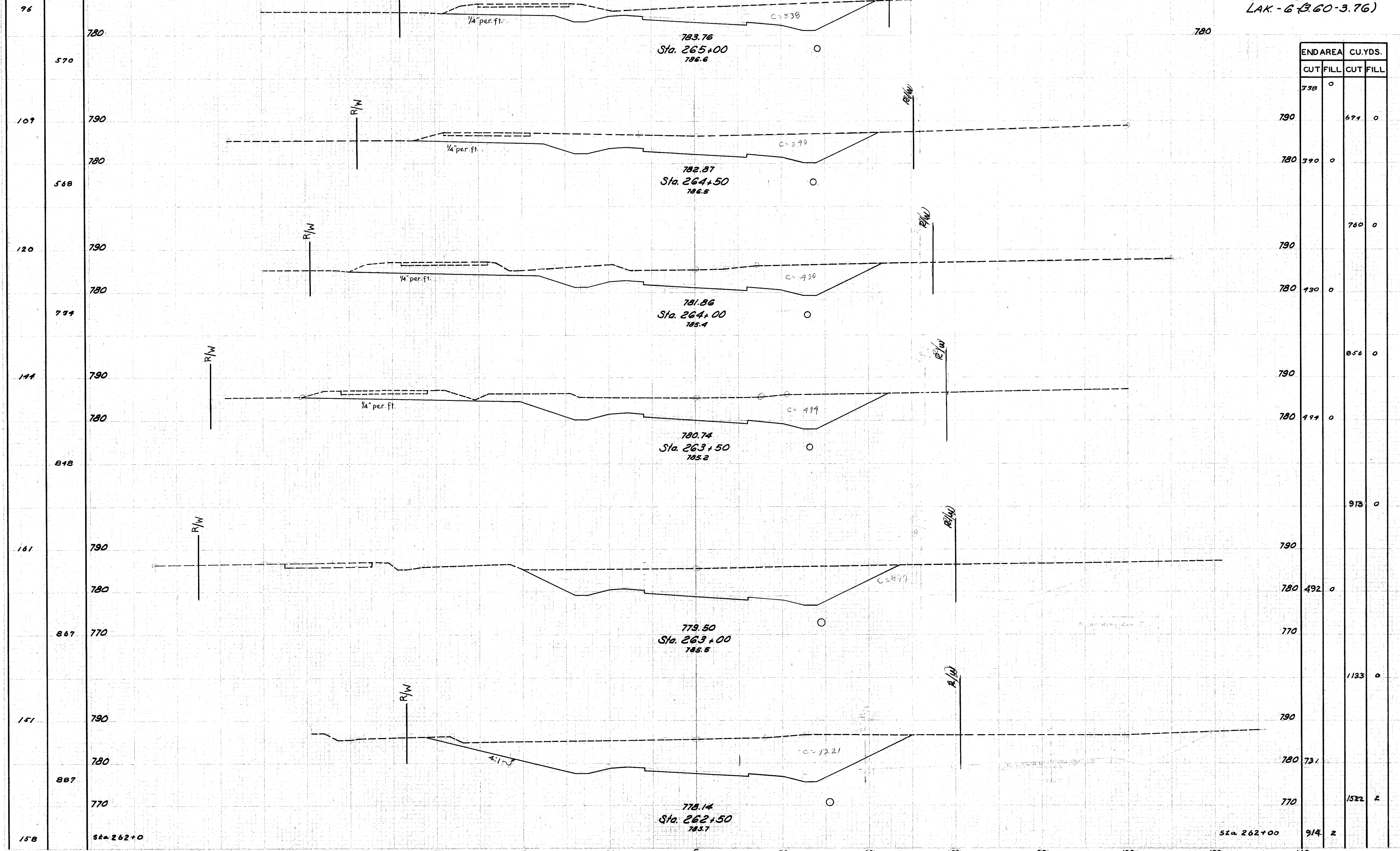
CROSS SECTIONS STA. 262+50 TO STA. 265+00
