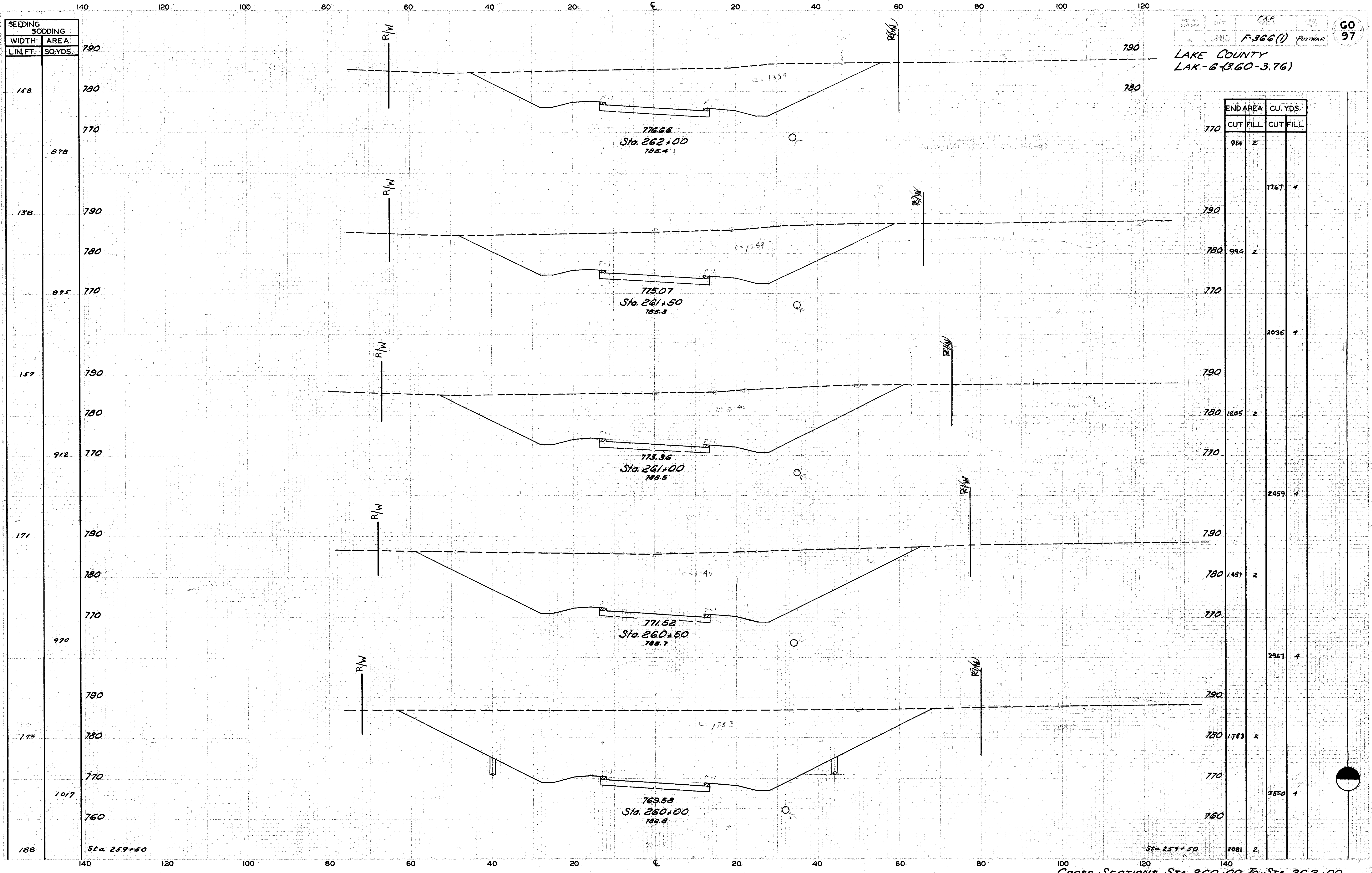
Cross Sections STA. 260+00 To STA. 262+00
