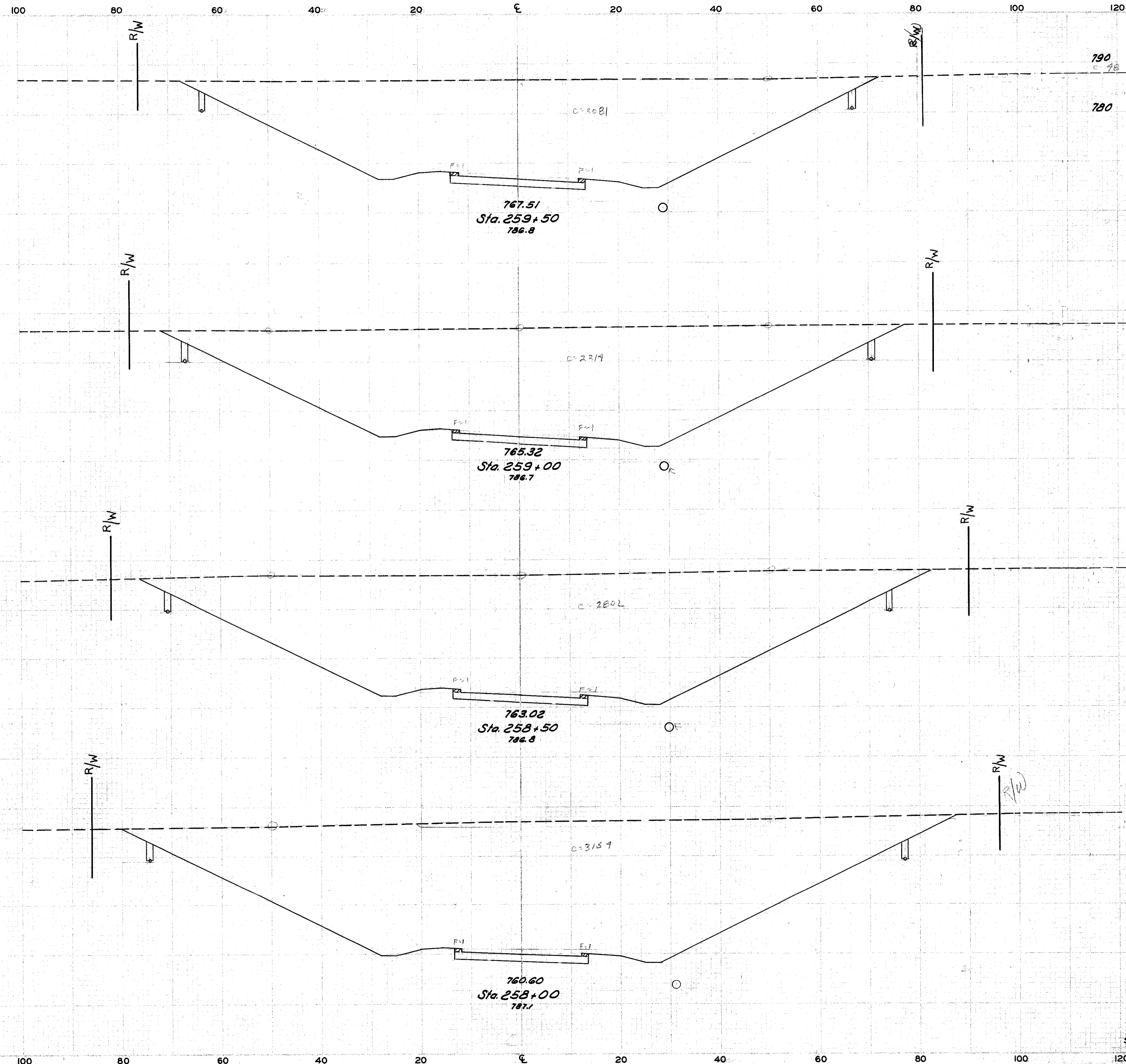
Cross Sections STA 258+00 TO STA 259+50
