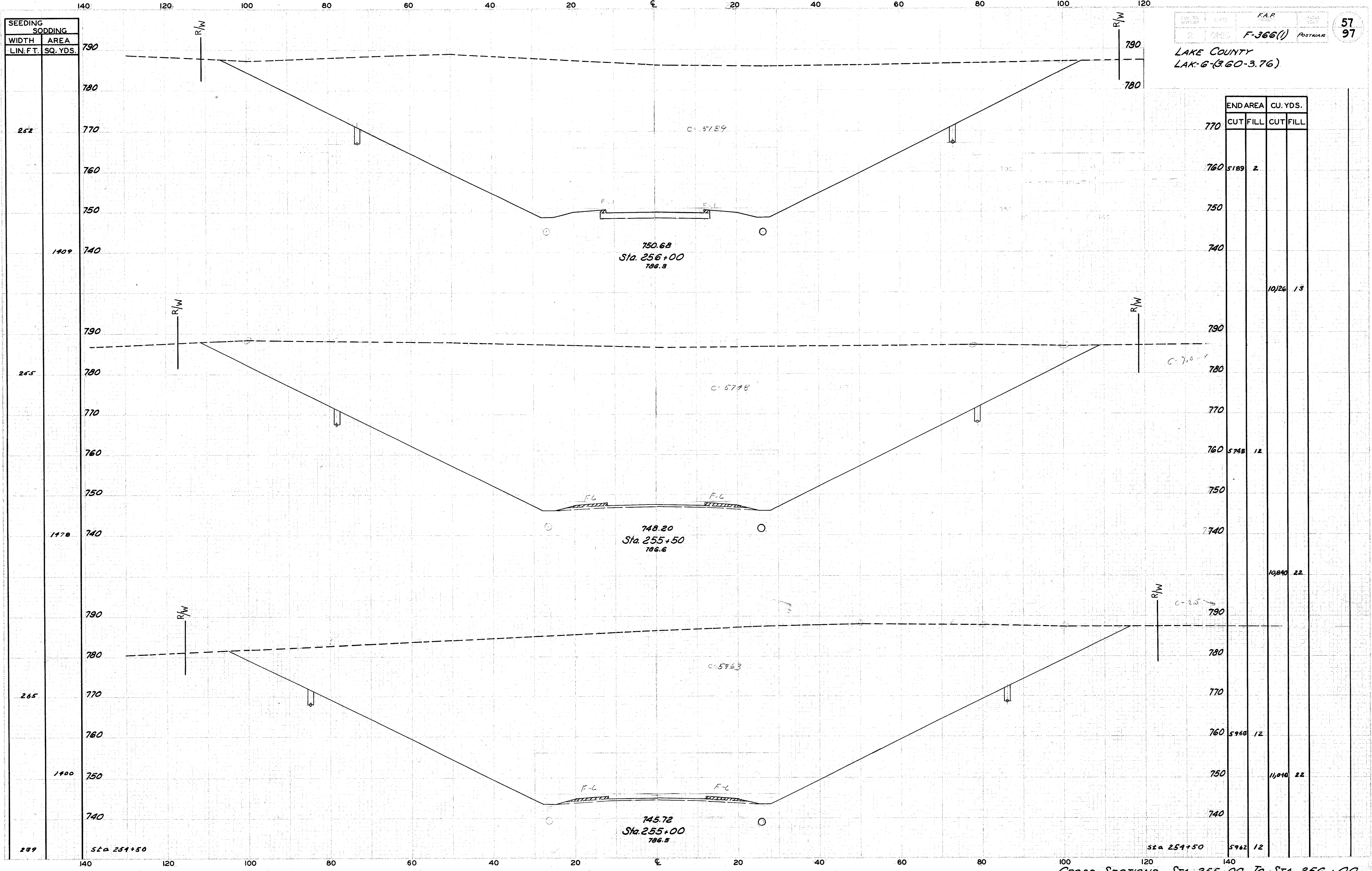
CROSS SECTIONS STA. 255+00 TO STA. 256+00
