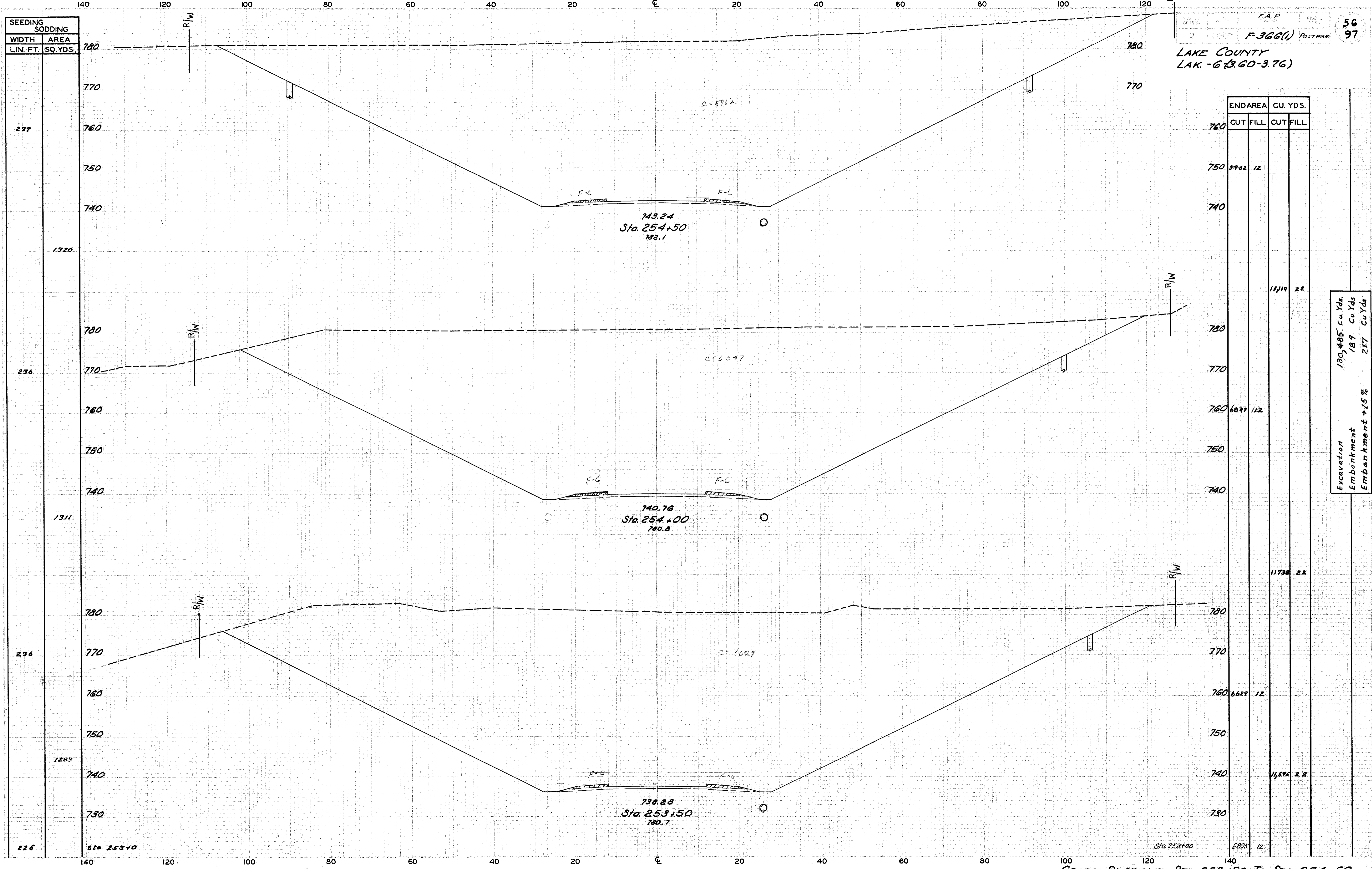
CROSS SECTIONS STA. 253+50 TO STA. 254+50
