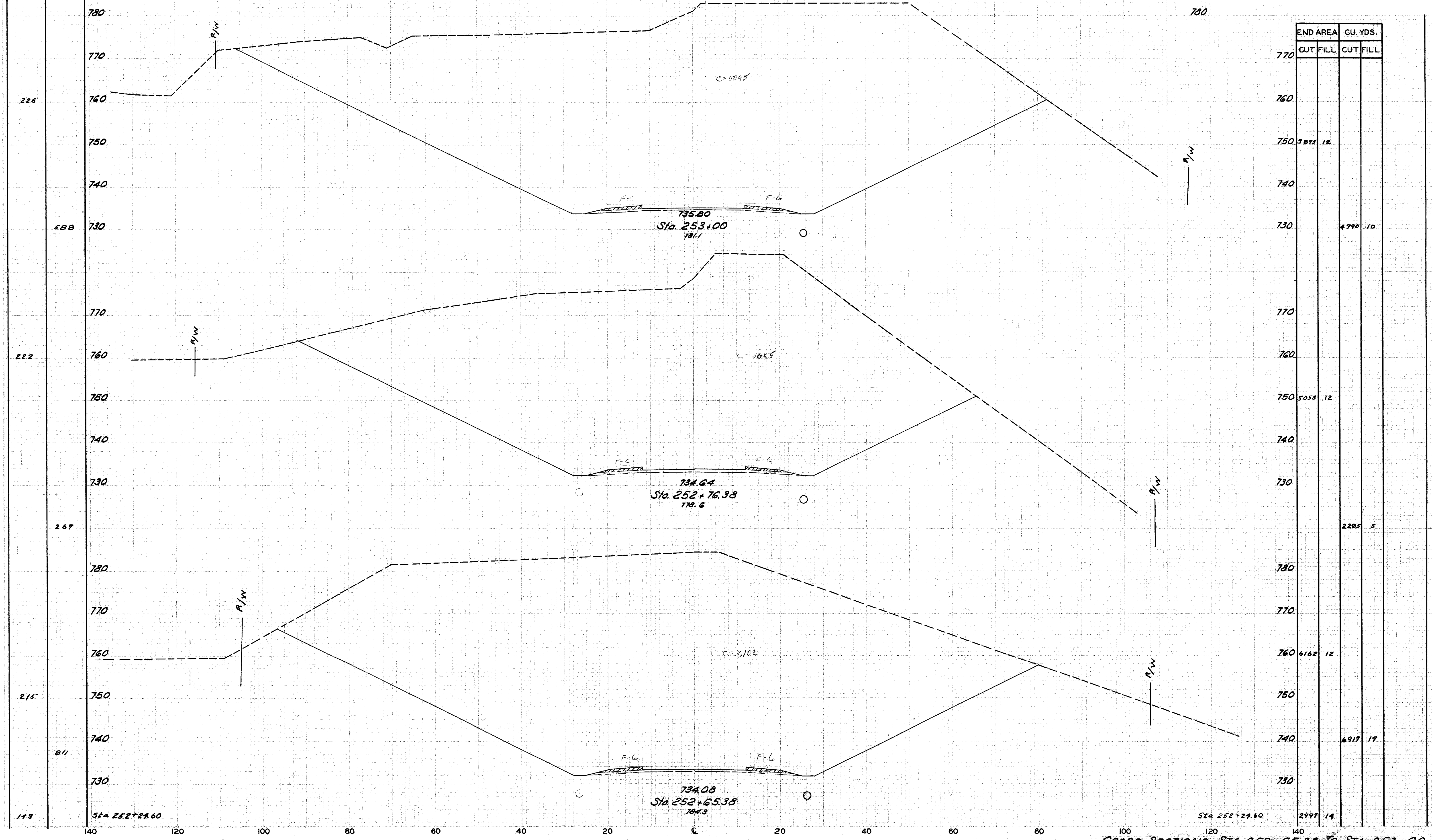
CROSS SECTIONS STA. 252+65.38 TO STA. 253+00
