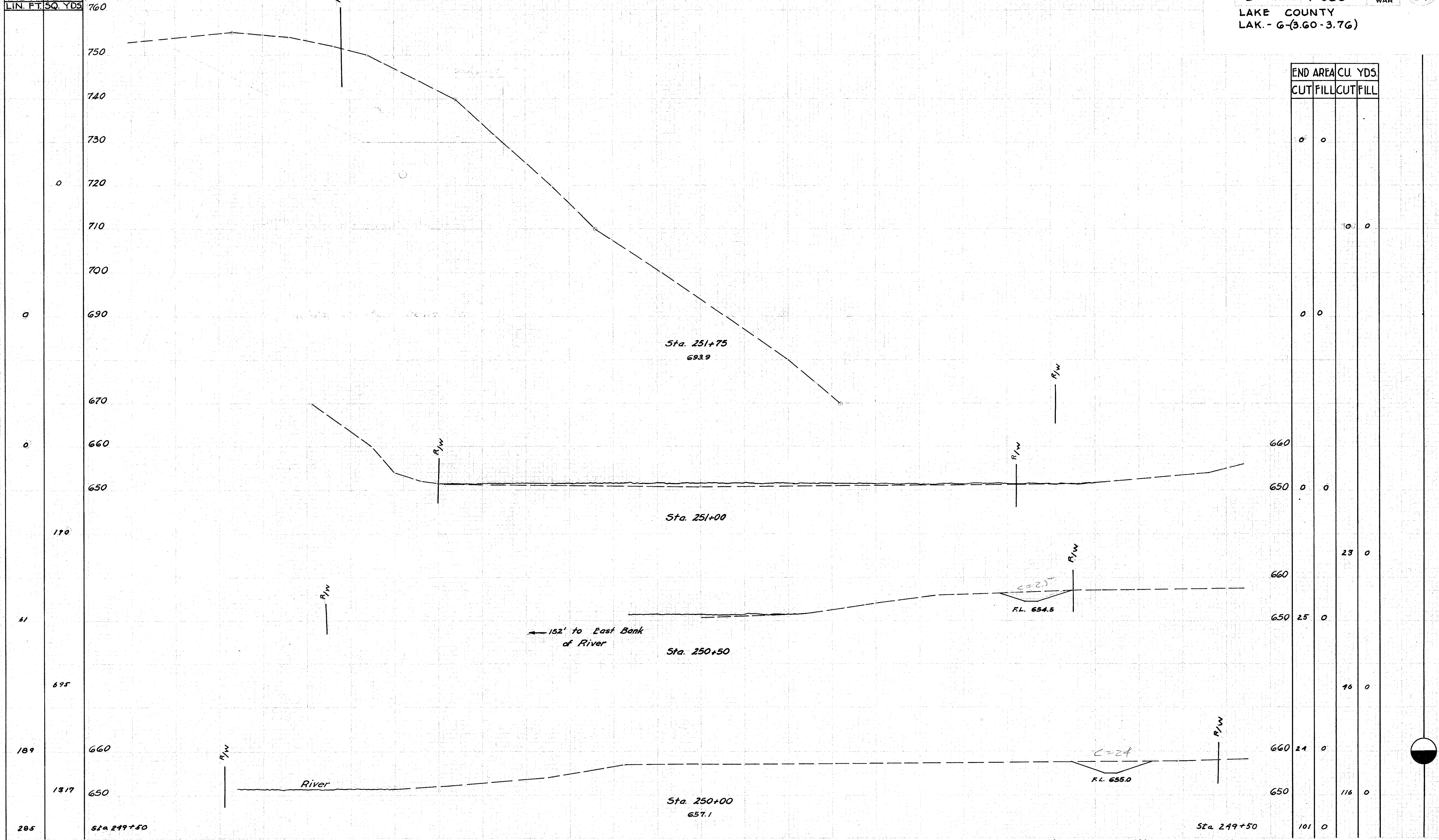
CROSS SECTIONS STA. 250+00 TO STA. 251+75
