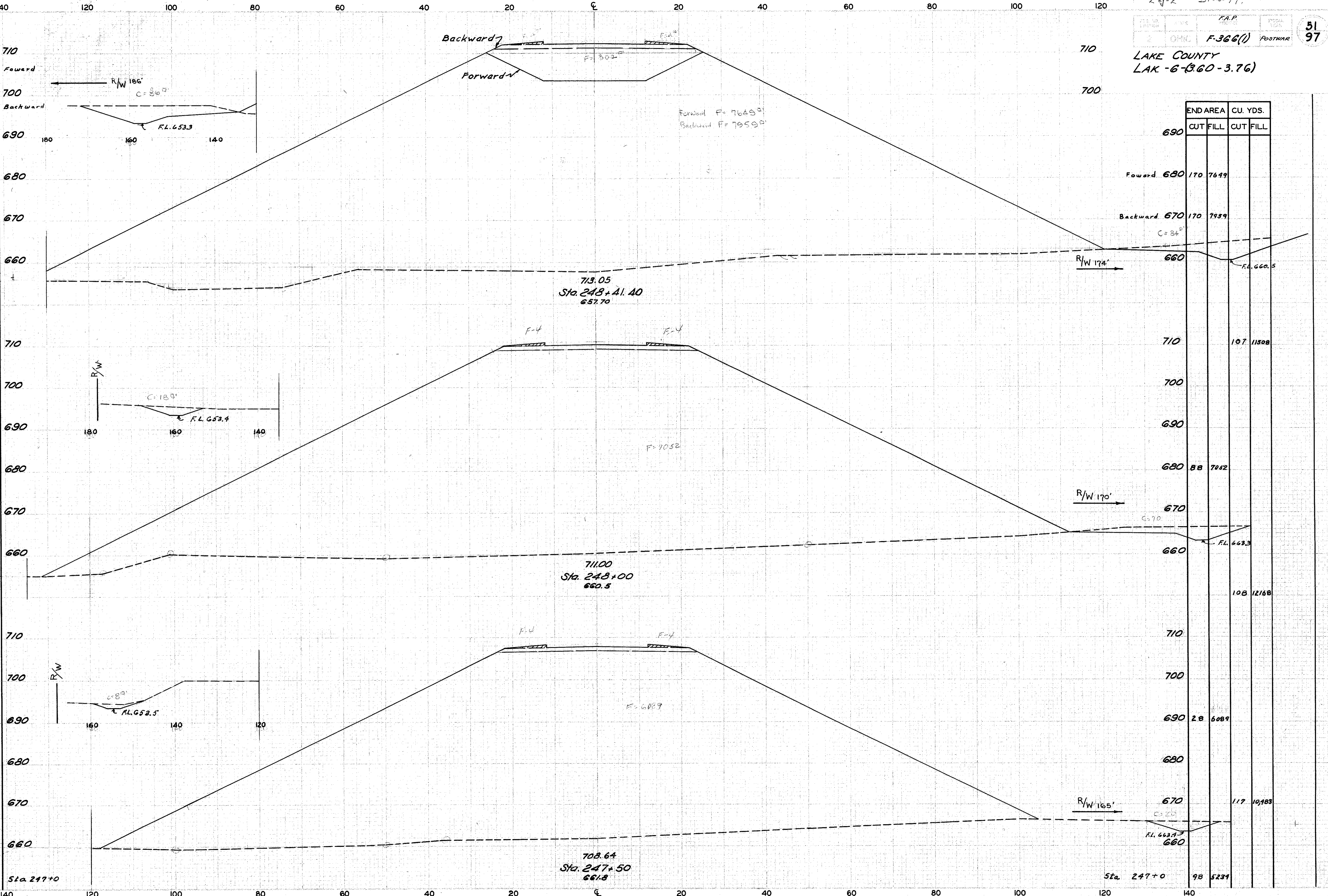
CROSS SECTIONS STA. 247+50 TO STA. 248+50
