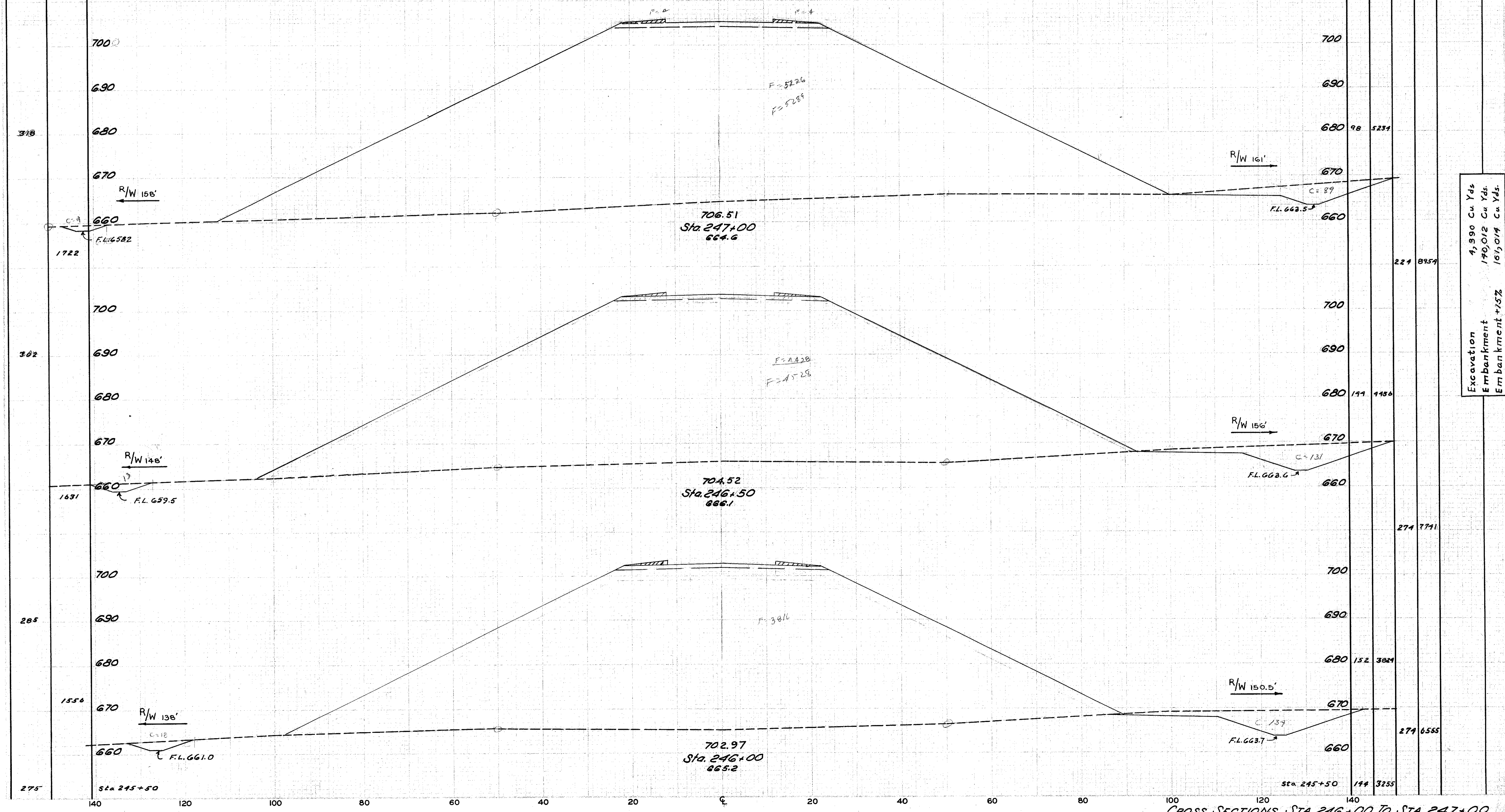
CROSS SECTIONS STA. 246+00 TO STA. 247+00
