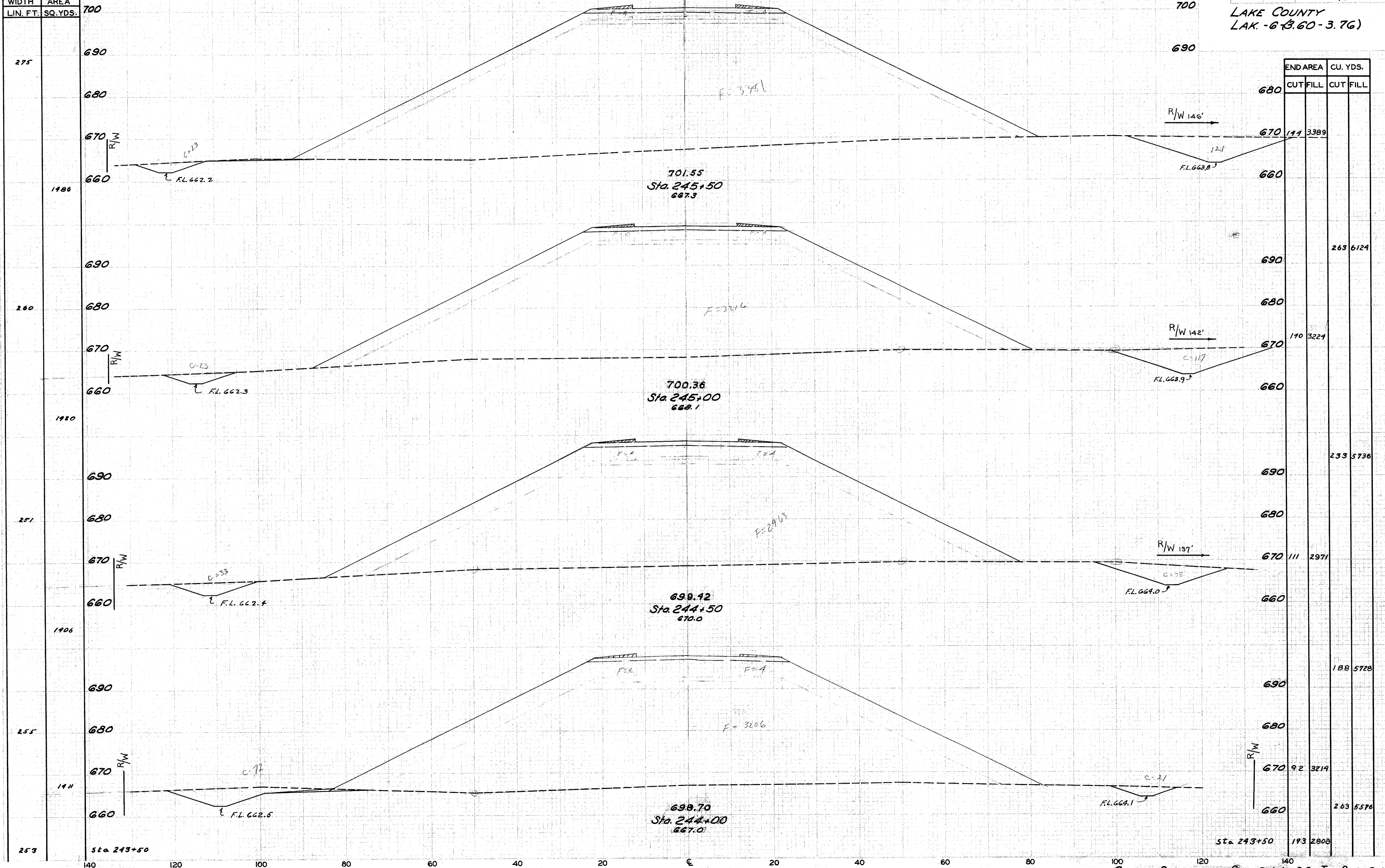
CROSS SECTIONS STA. 244+00 TO STA. 245+50
