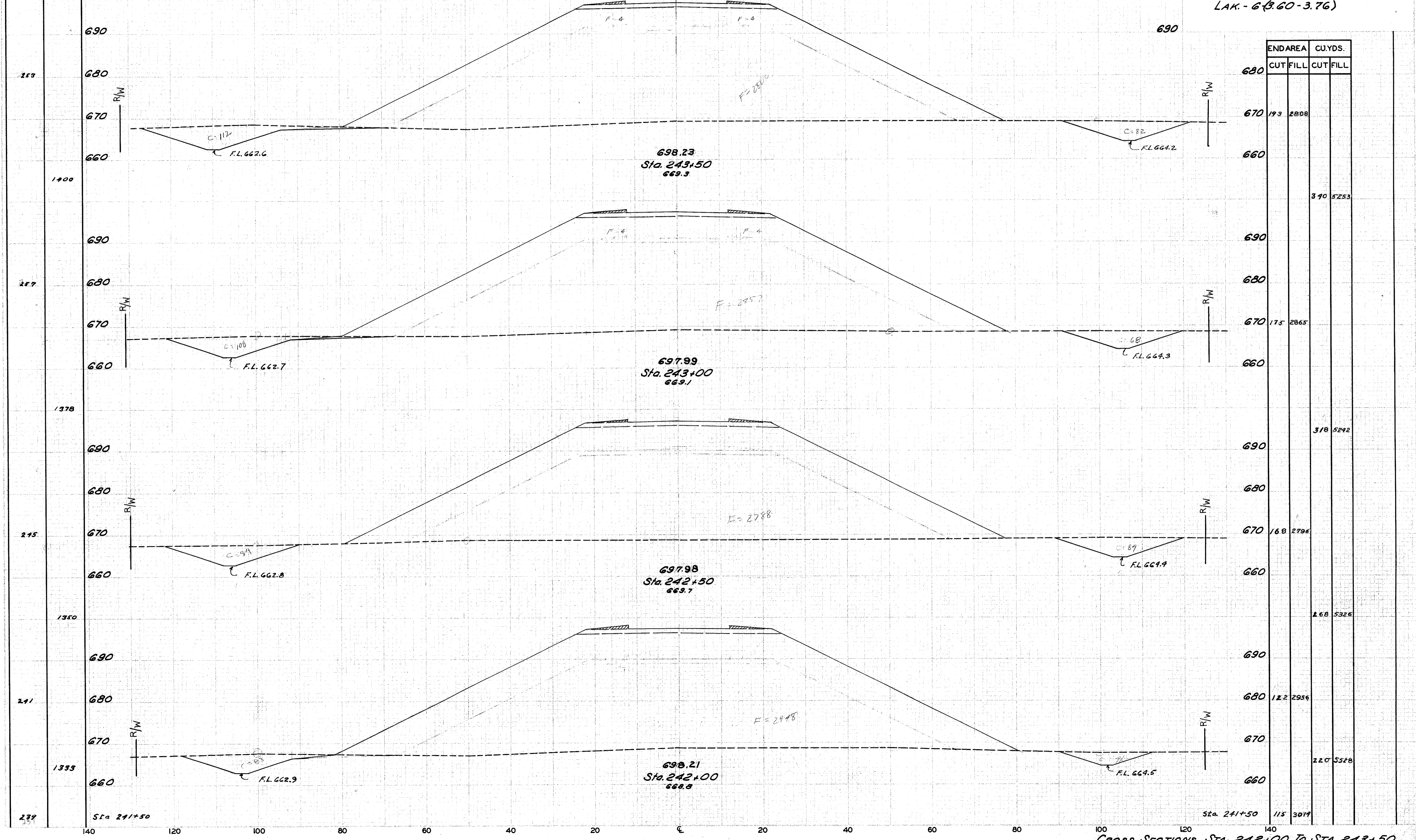
Cross Sections Sta. 242+00 To Sta. 243+50
