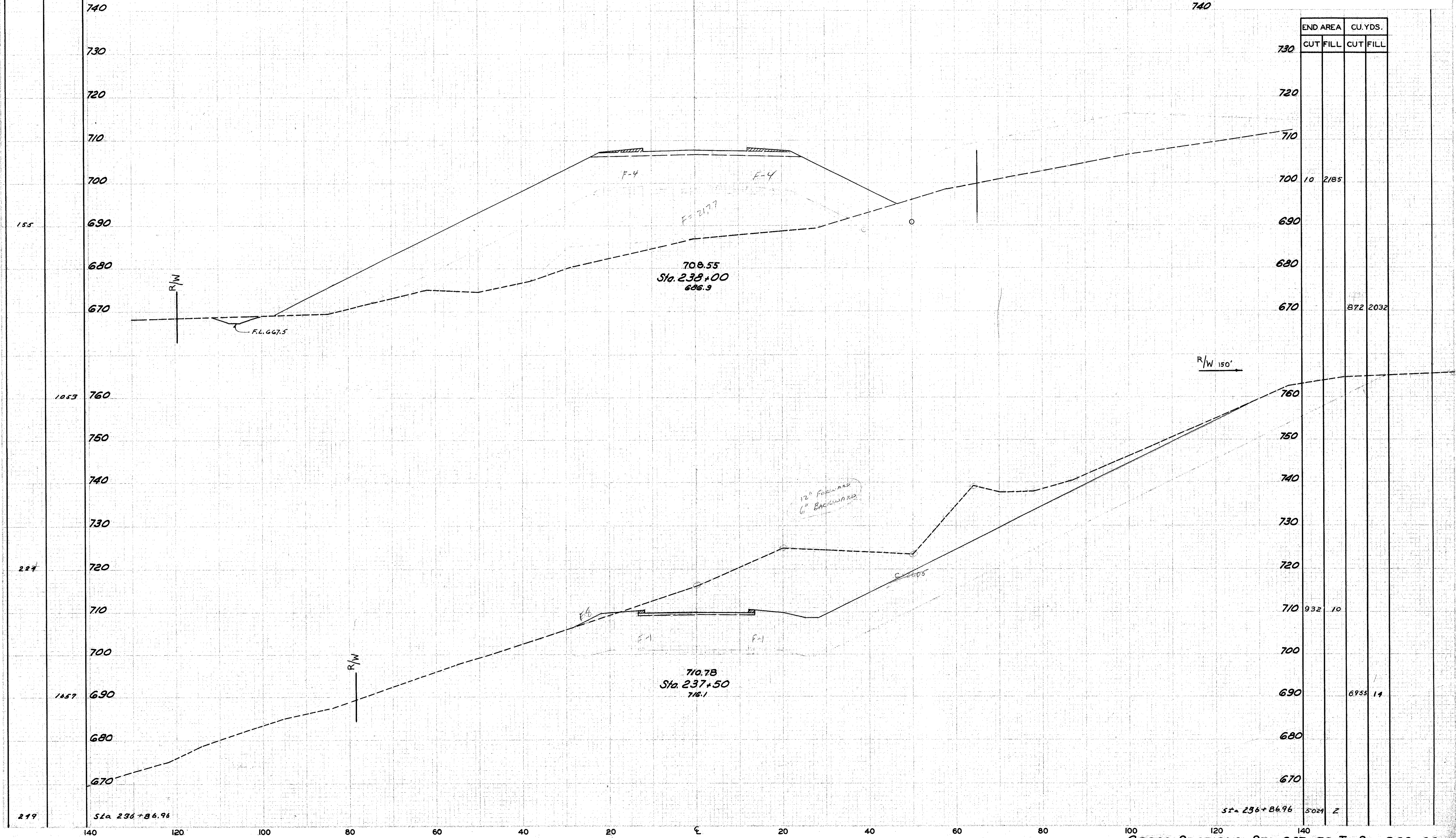
CROSS SECTIONS STA. 237+50 TO STA. 238+00
