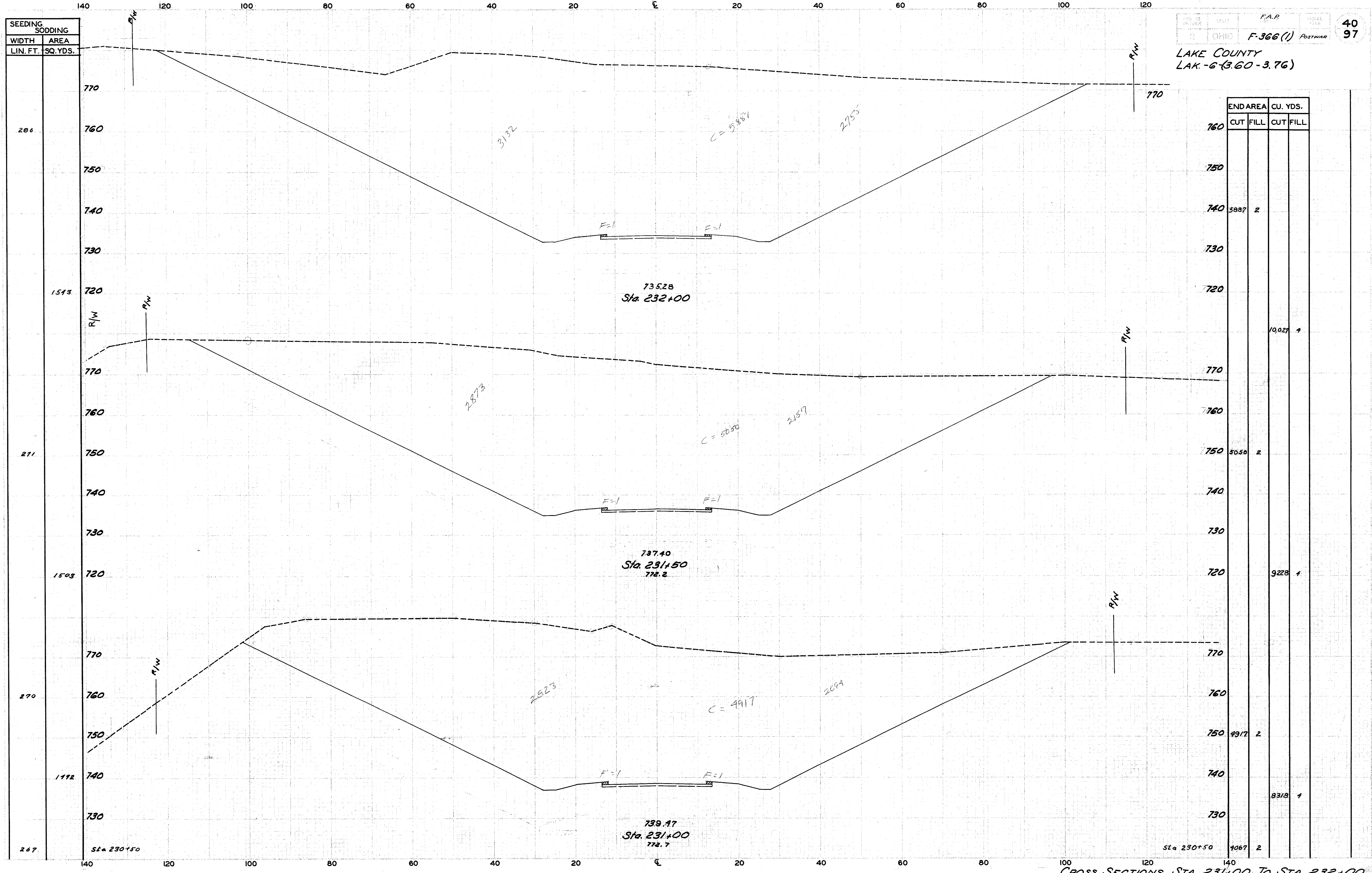
CROSS SECTIONS STA. 231+00 TO STA. 232+00
