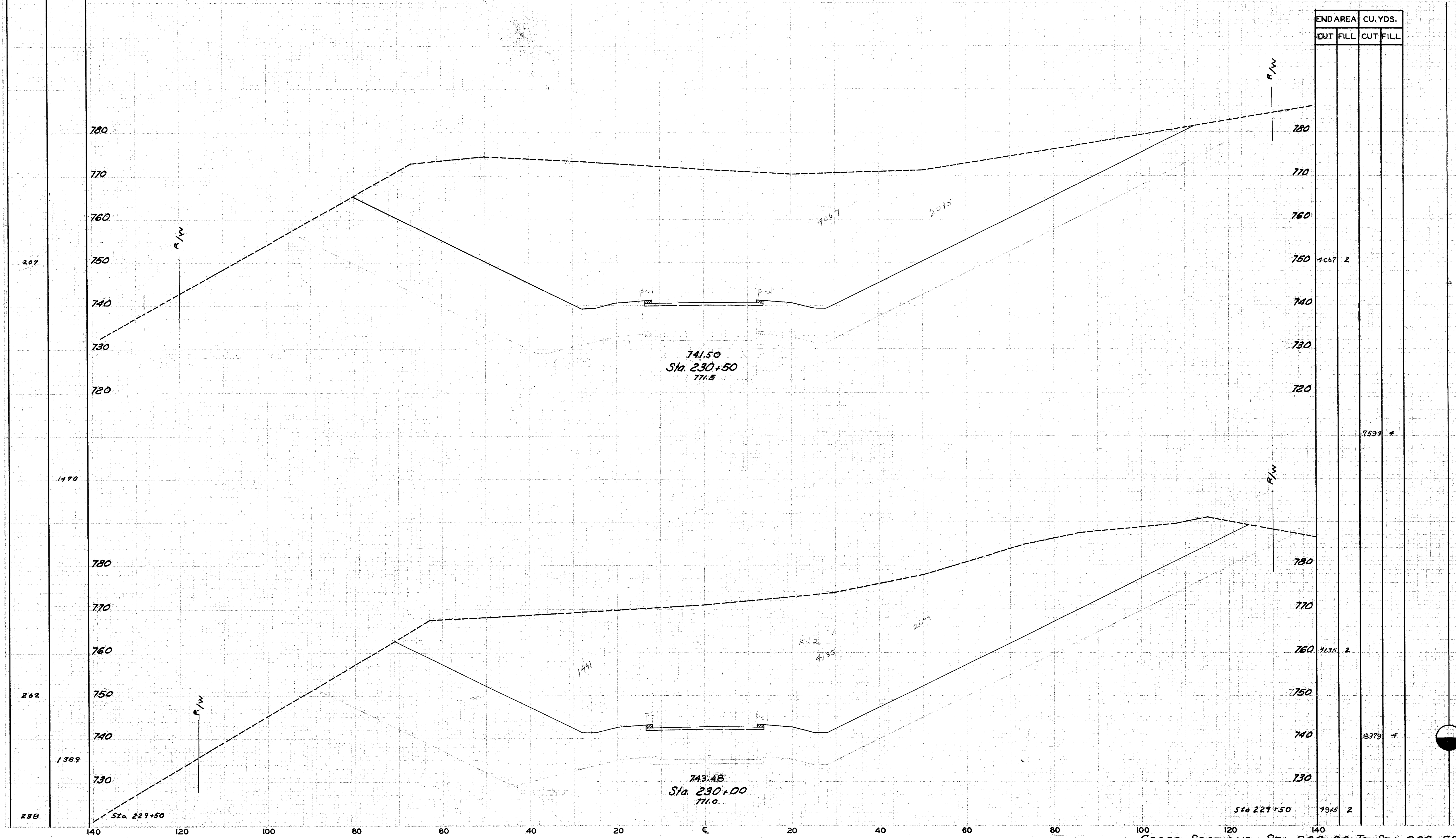
CROSS SECTIONS STA. 230+00 TO STA. 230+50
