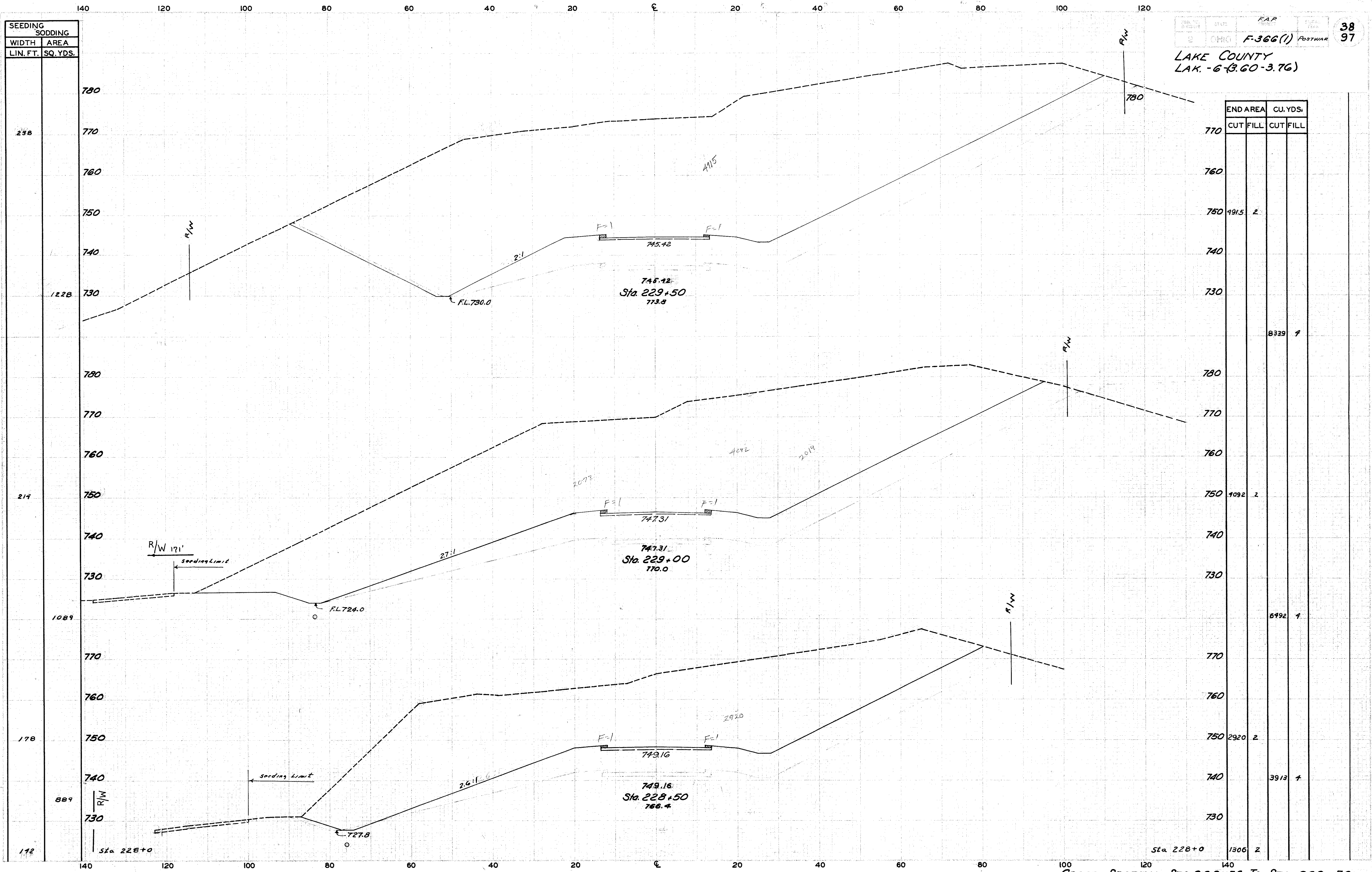
Cross Section STA. 228+50 TO STA. 229+50
