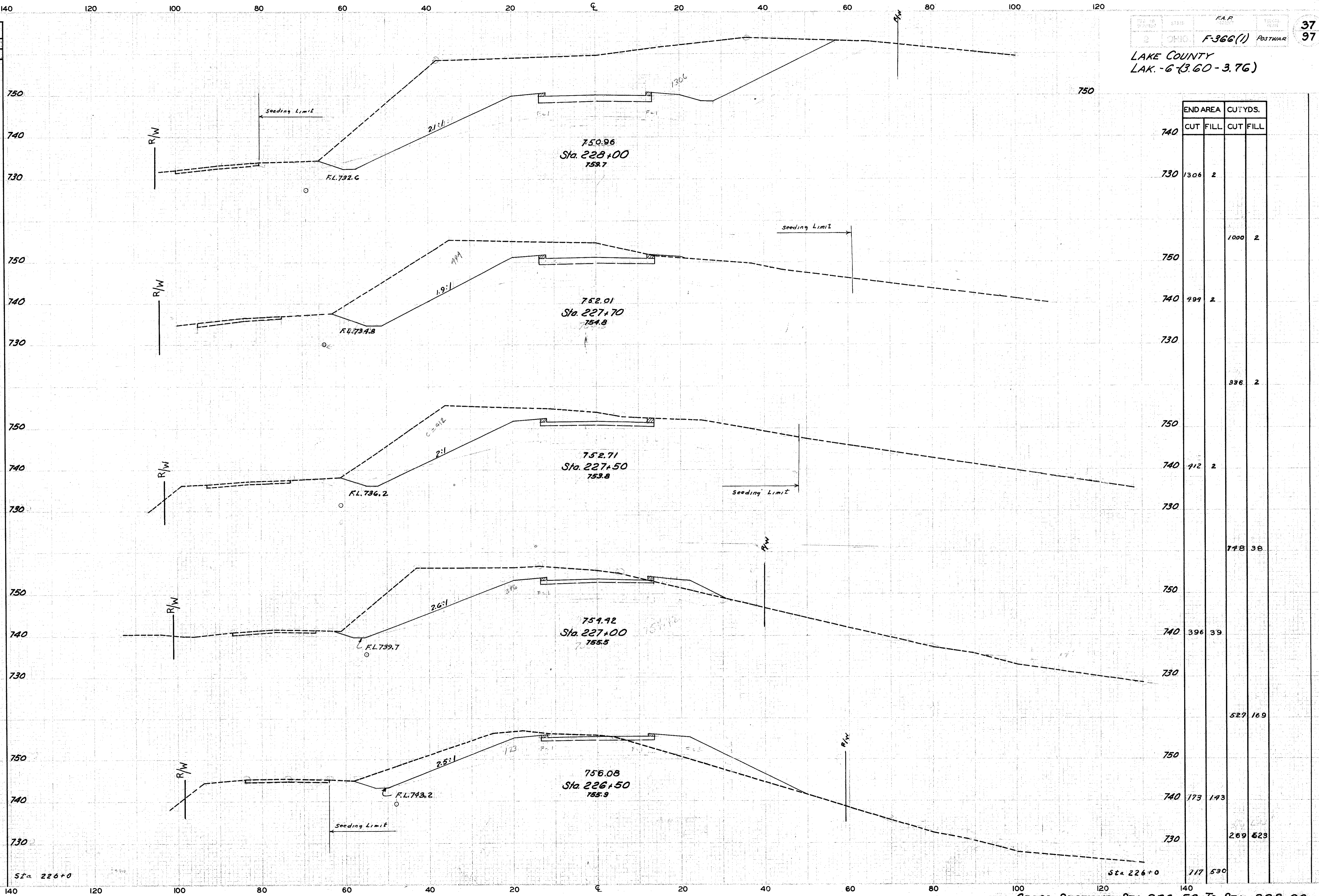
CROSS SECTIONS STA. 226+50 TO STA. 228+00
