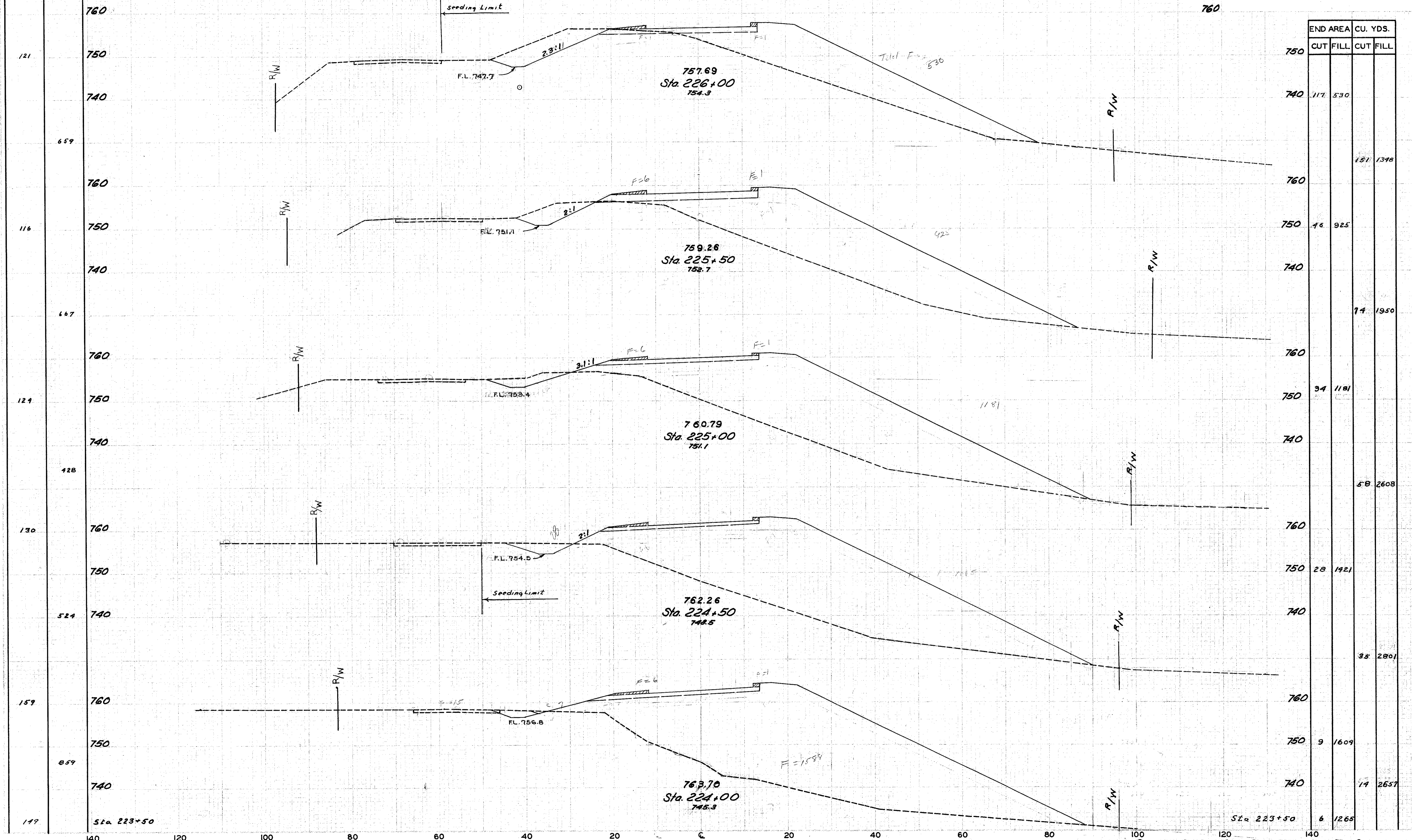
CROSS SECTIONS STA. 224+00 TO STA. 226+00
