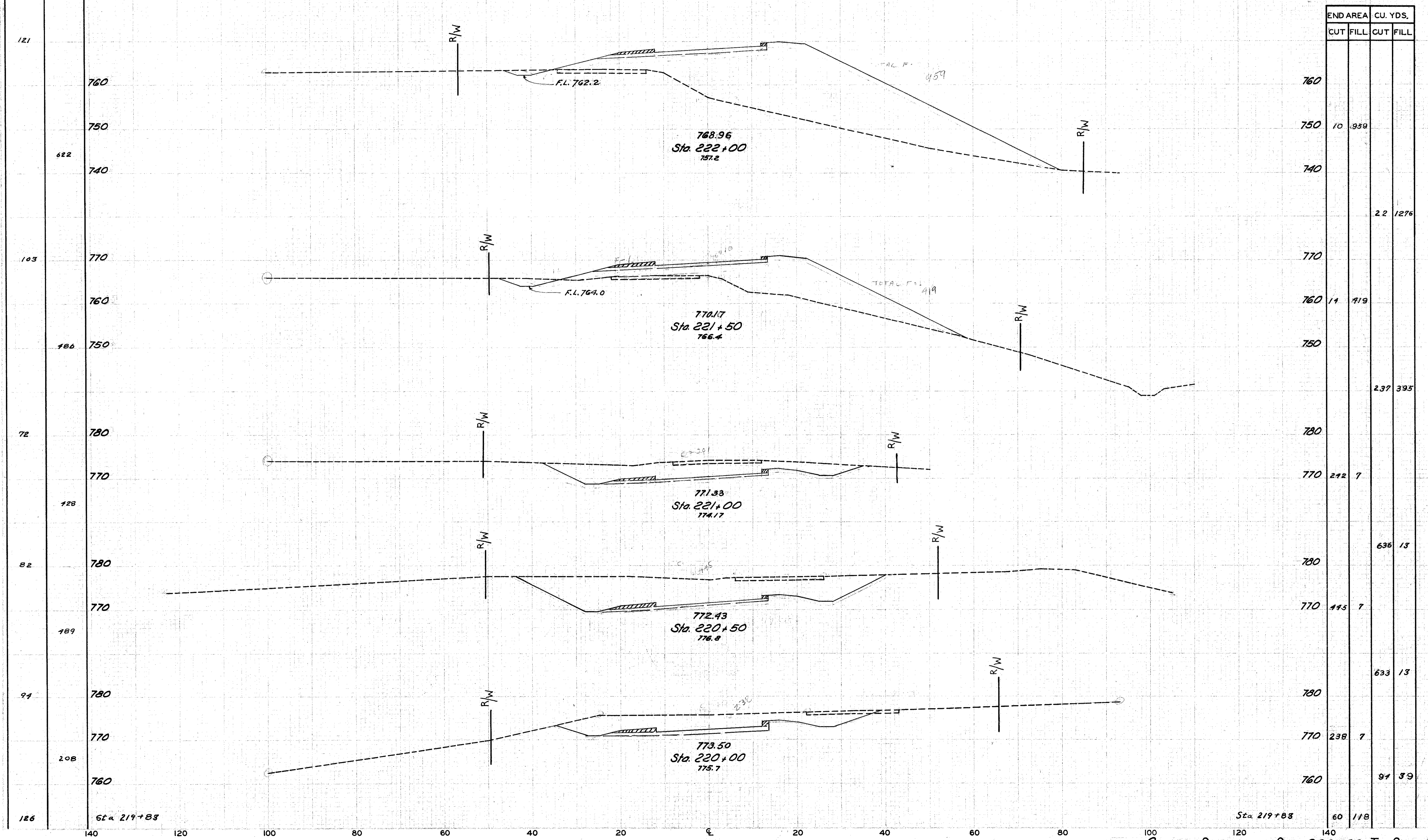
CROSS SECTIONS STA. 220+00 TO STA. 222+00
