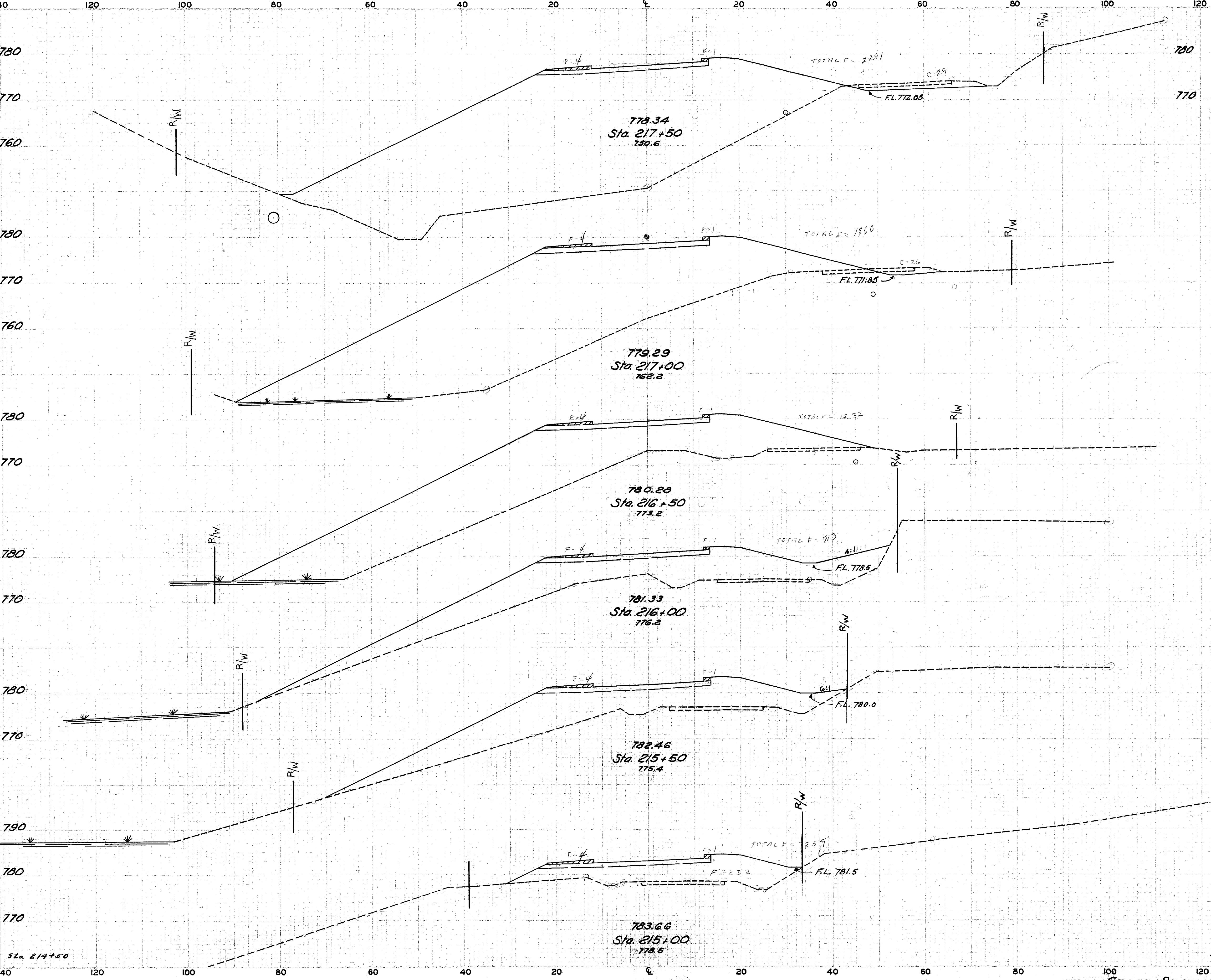
CROSS SECTIONS STA. 215+00 TO STA. 217+50
