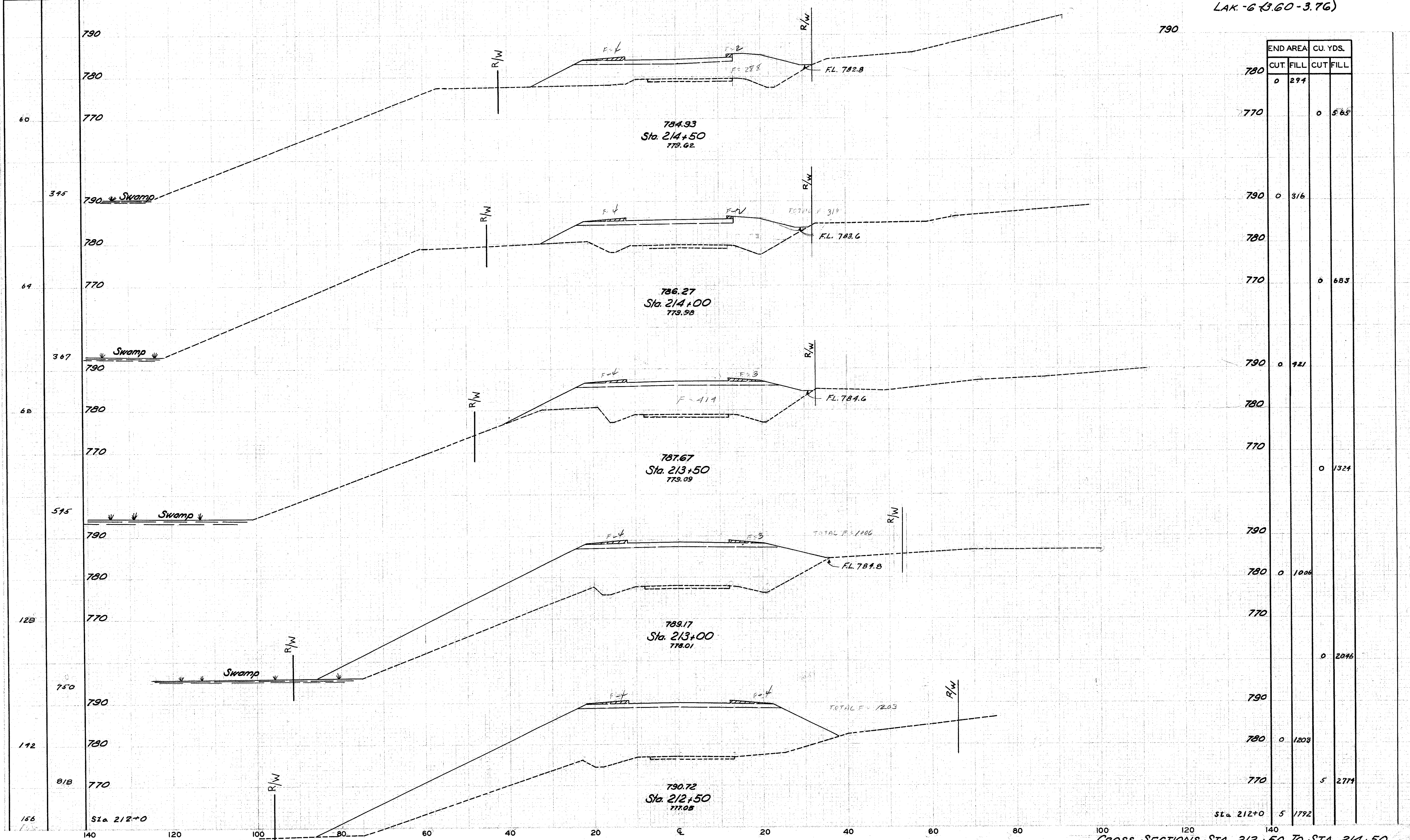
CROSS SECTIONS STA. 212+50 TO STA. 214+50
