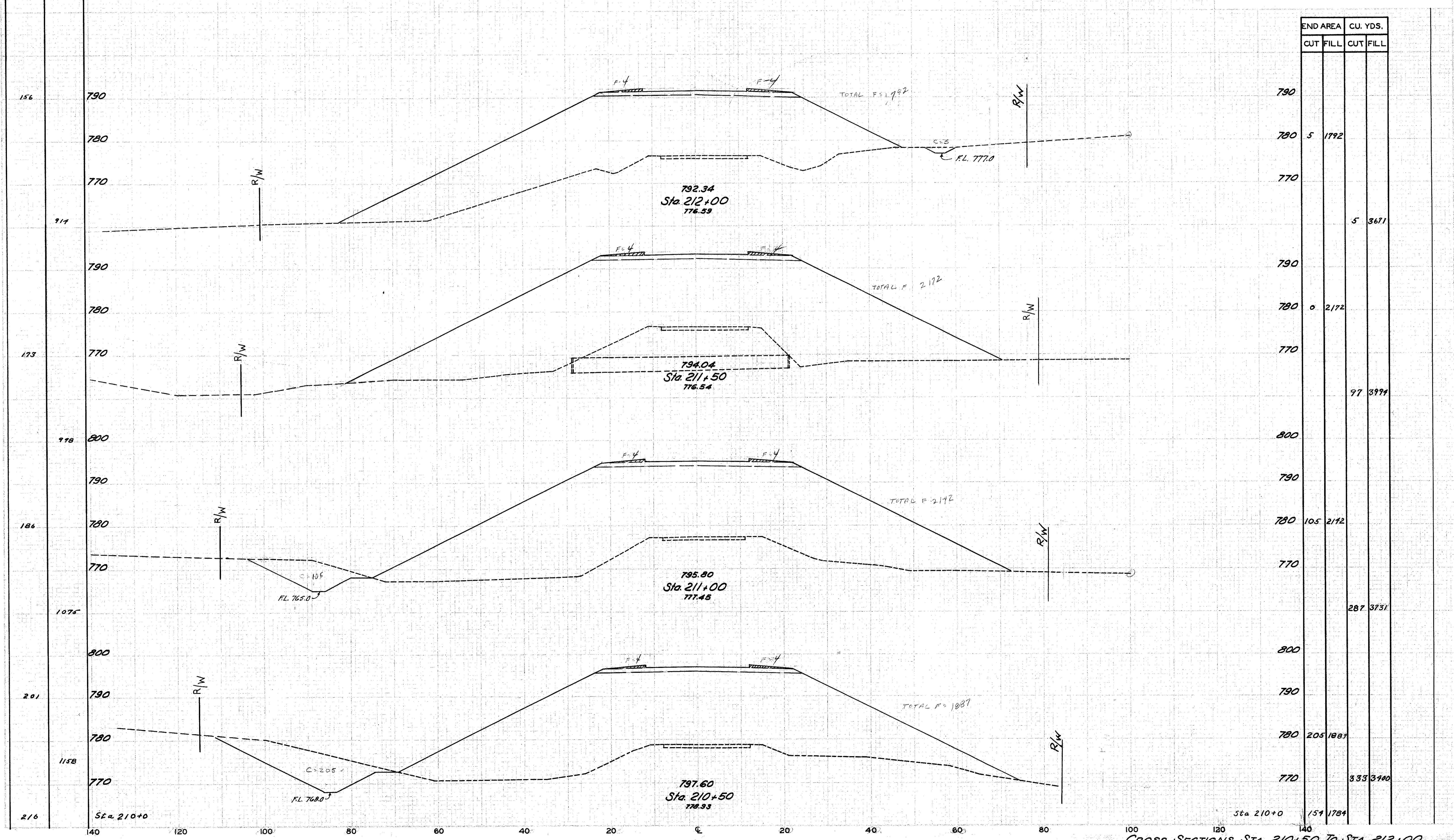
CROSS SECTIONS STA. 210+50 TO STA. 212+00
