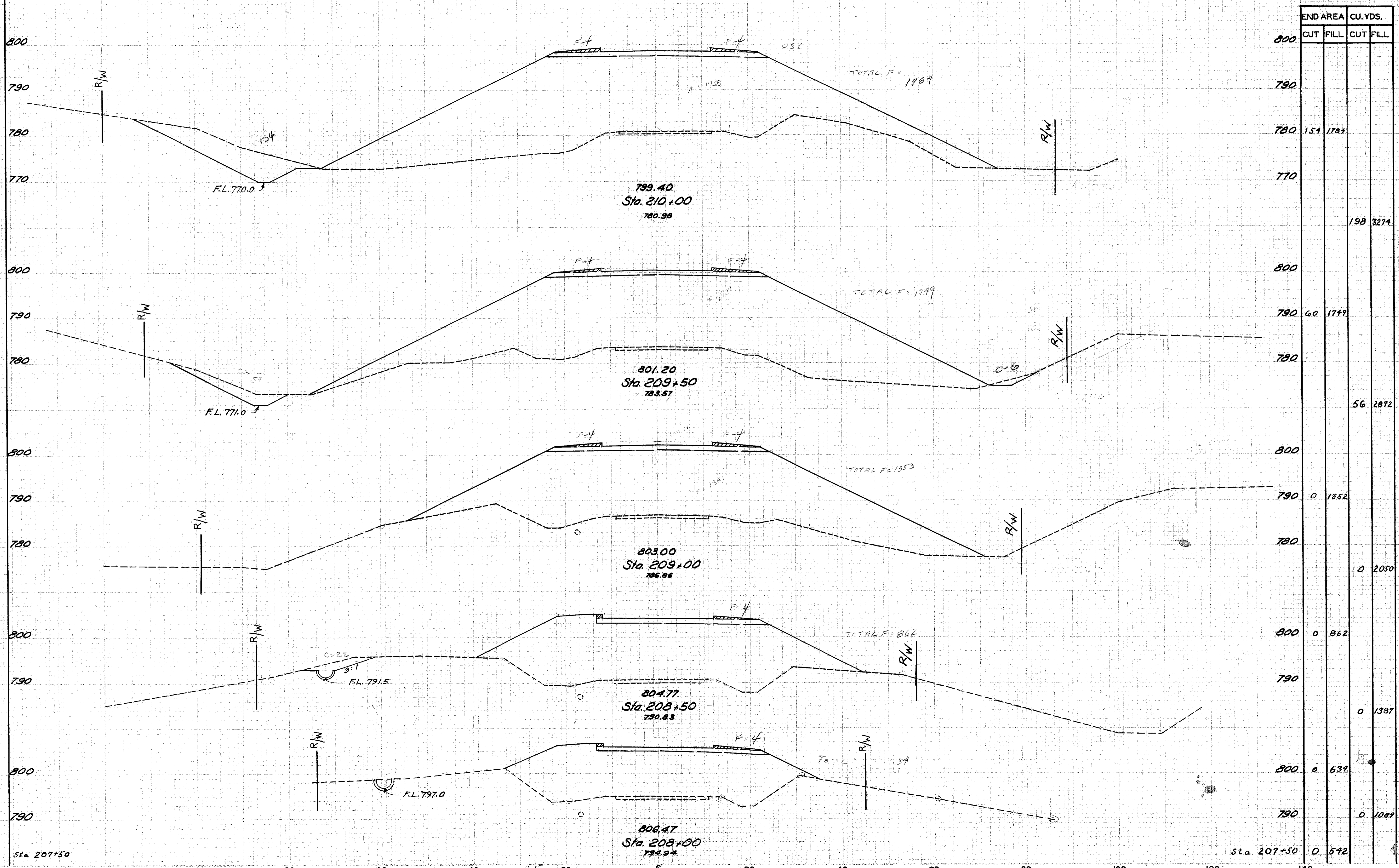
CROSS SECTIONS STA. 208+00 TO STA. 210+00
