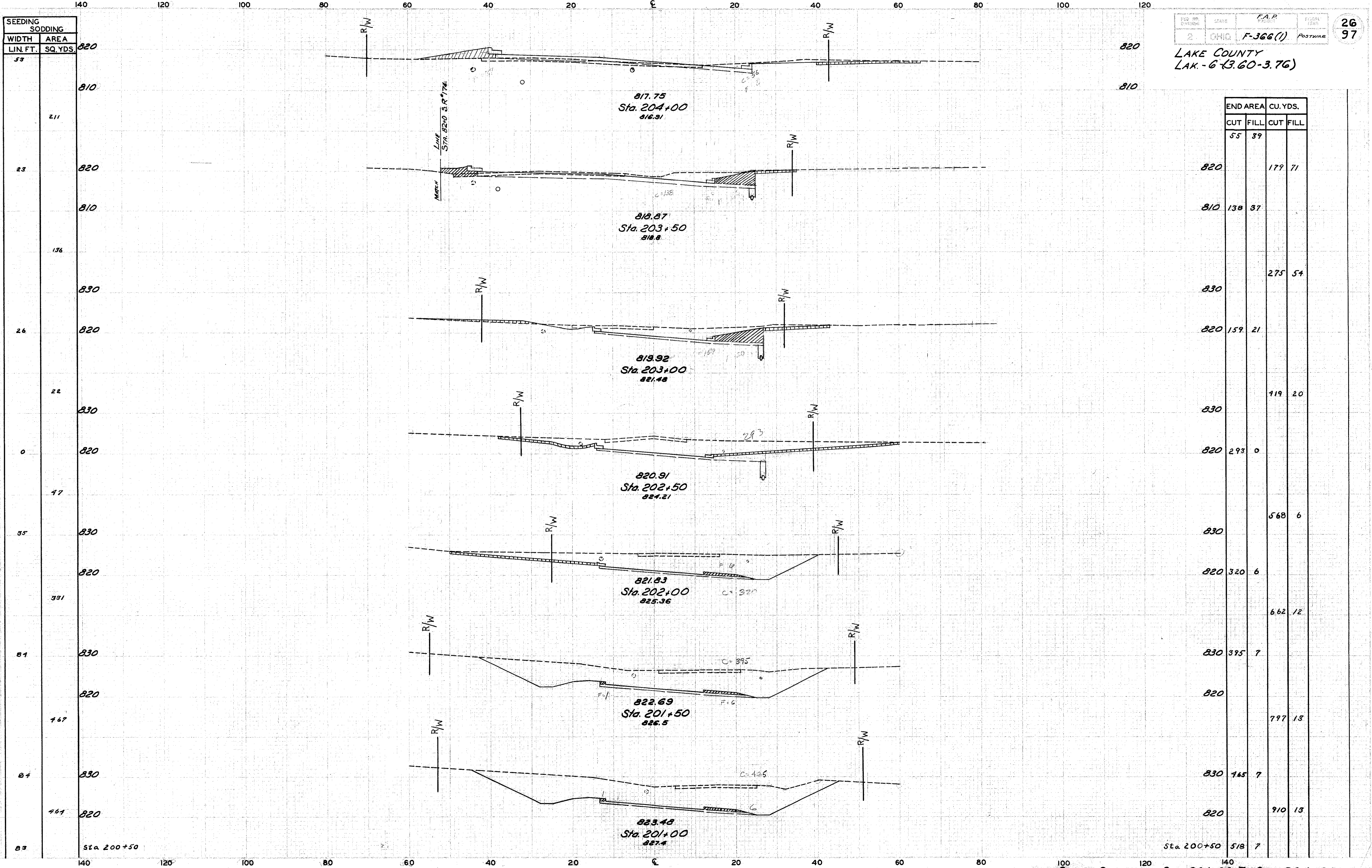
Cross SECTIONS STA. 201+00 TO STA. 204+00
