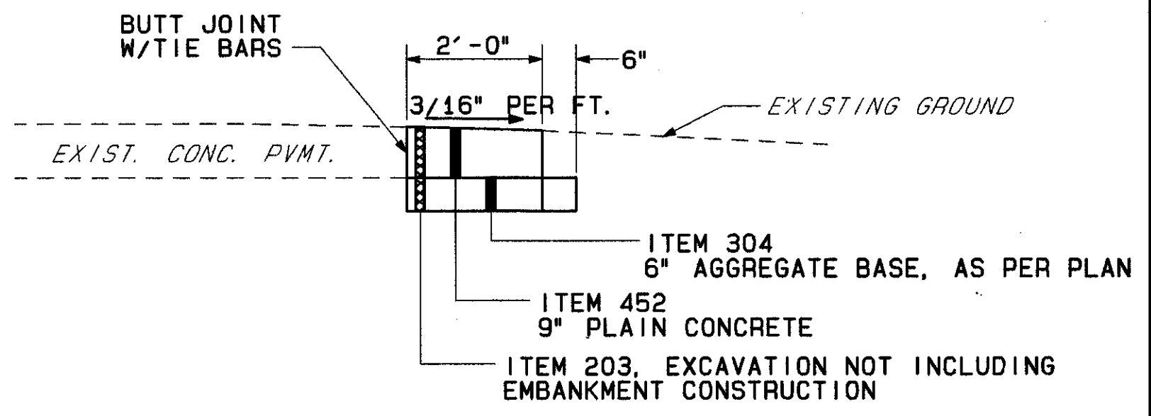
SECT. A-A STA. 47+60.40 TO STA. 49+55.15
