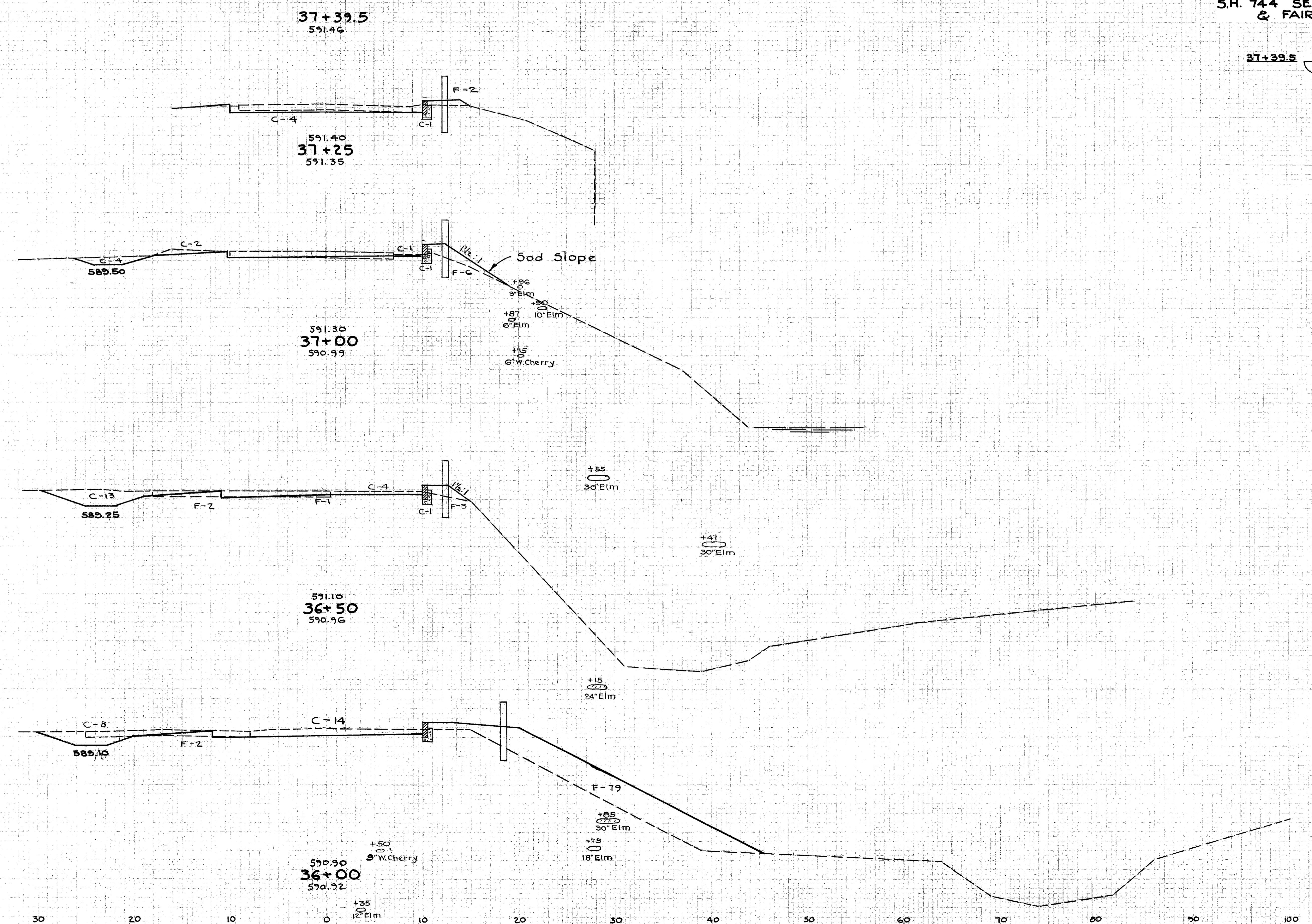
CROSS SECTIONS STA. 36+00 To STA. 37+39.5
