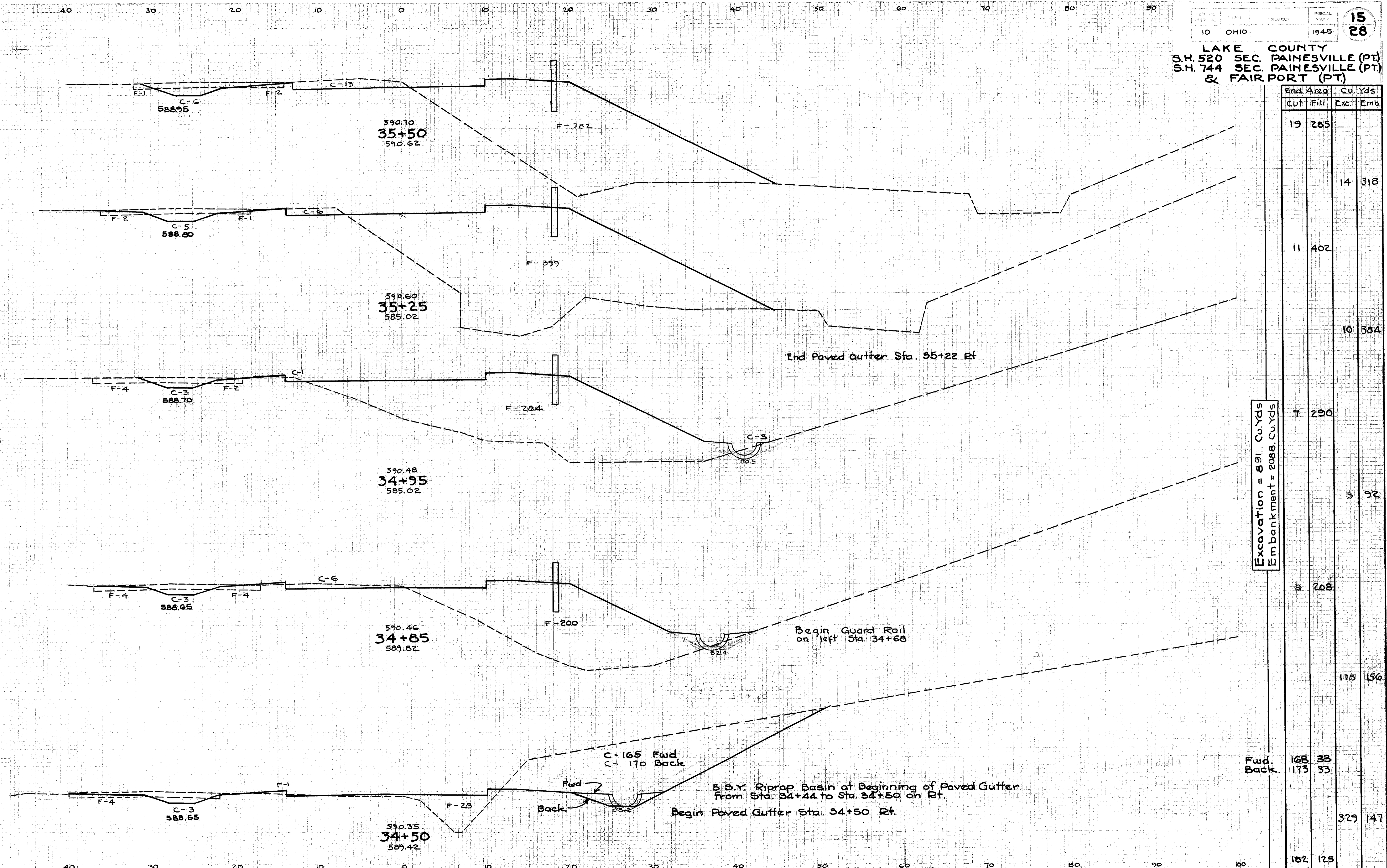
CROSS SECTIONS STA. 34+50 TO STA. 35+50
