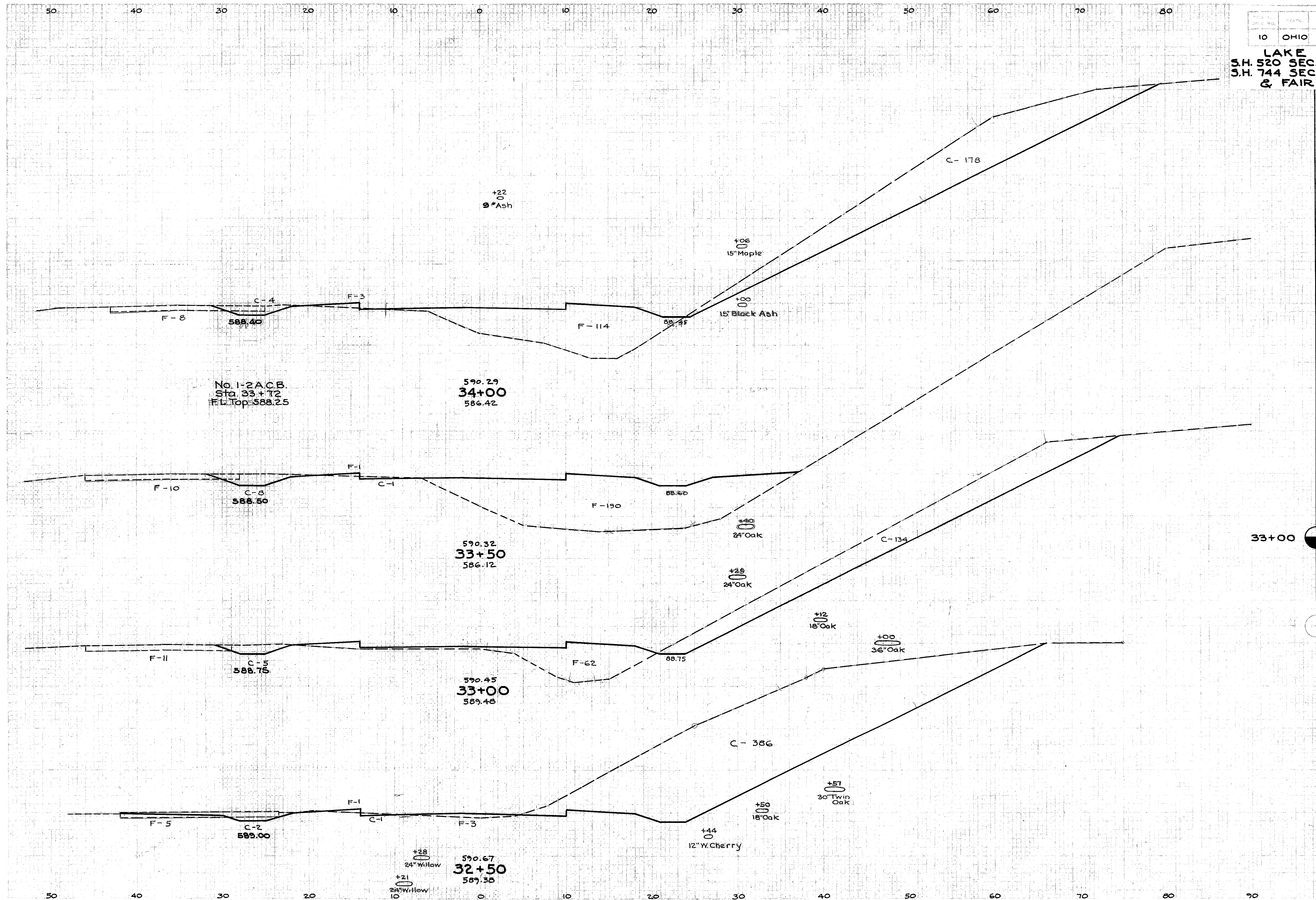
CROSS SECTIONS STA. 32+50 TO STA. 34+00
