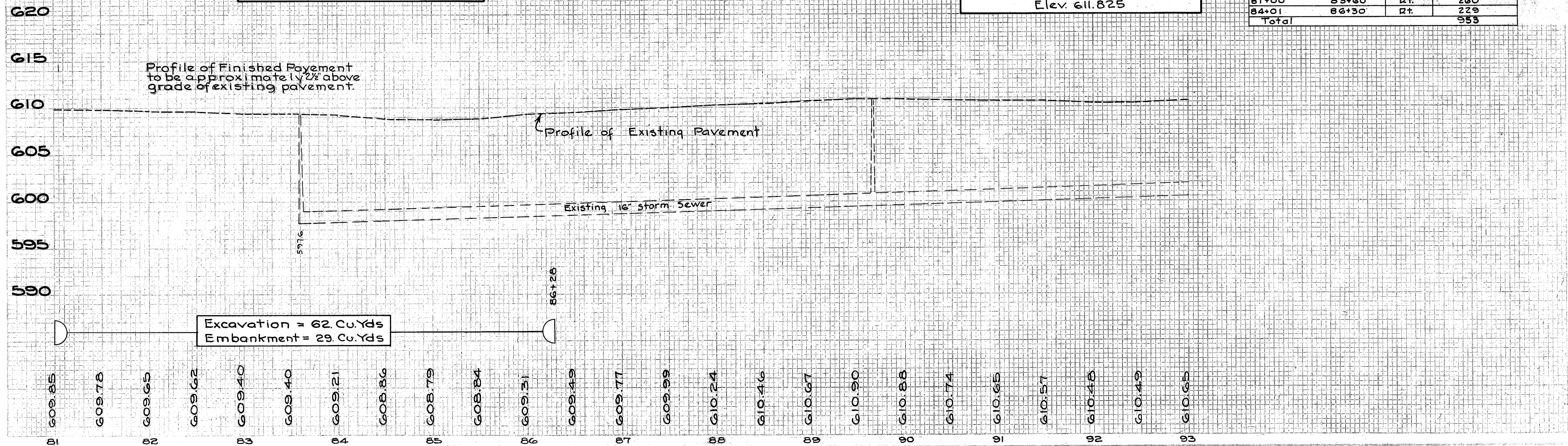
PLAN & PROFILE STA. 81+00 TO STA. 93+00
