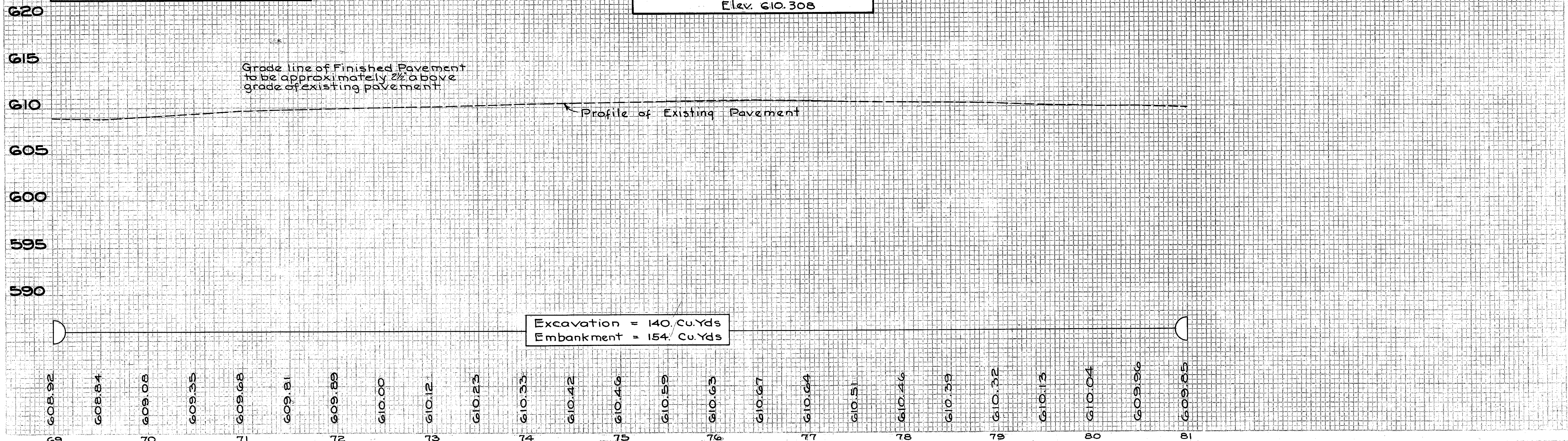
PLAN & PROFILE STA. 69+00 TO STA. 81+00
