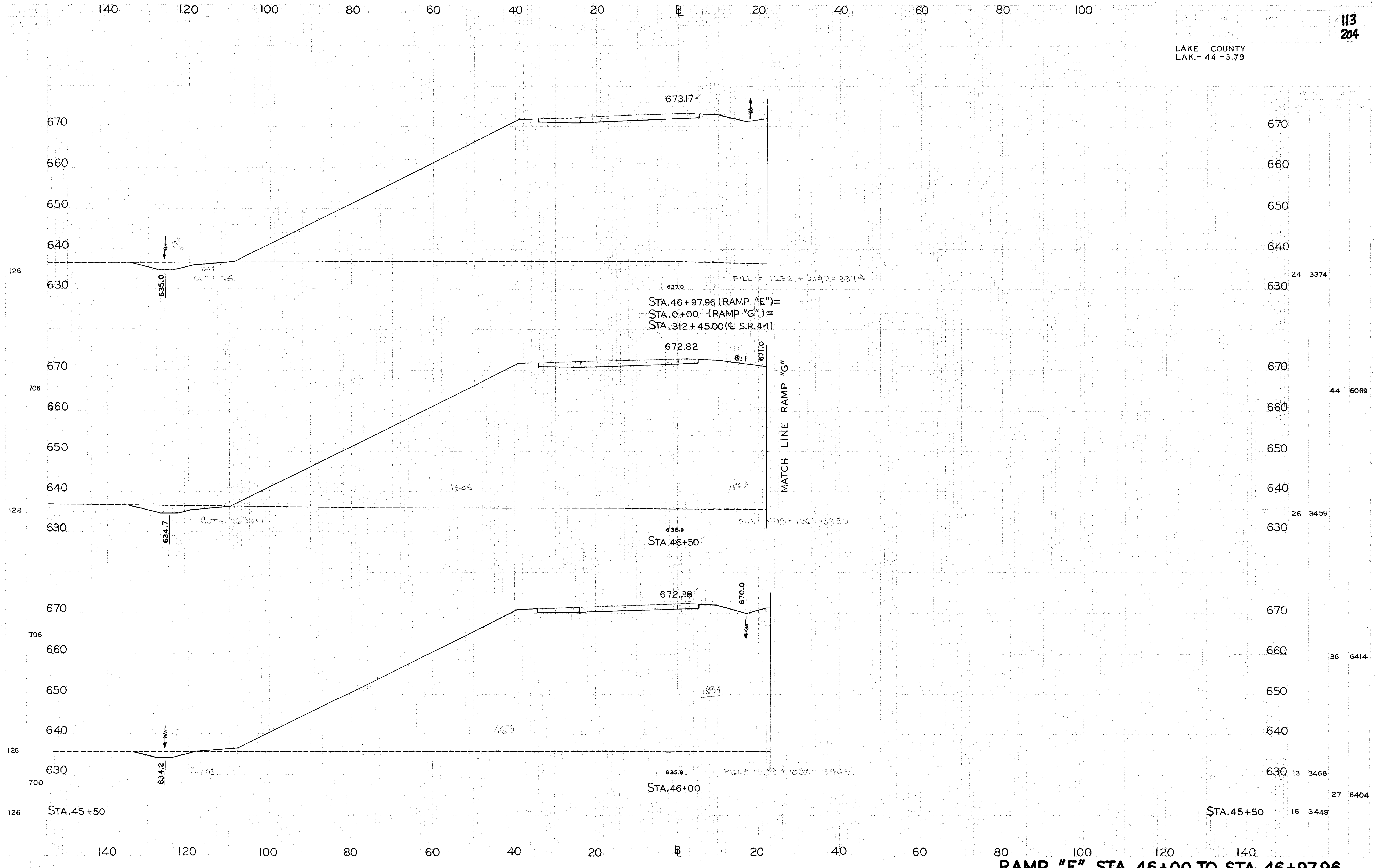
RAMP "E" STA. 46+00 TO STA. 46+97.96
