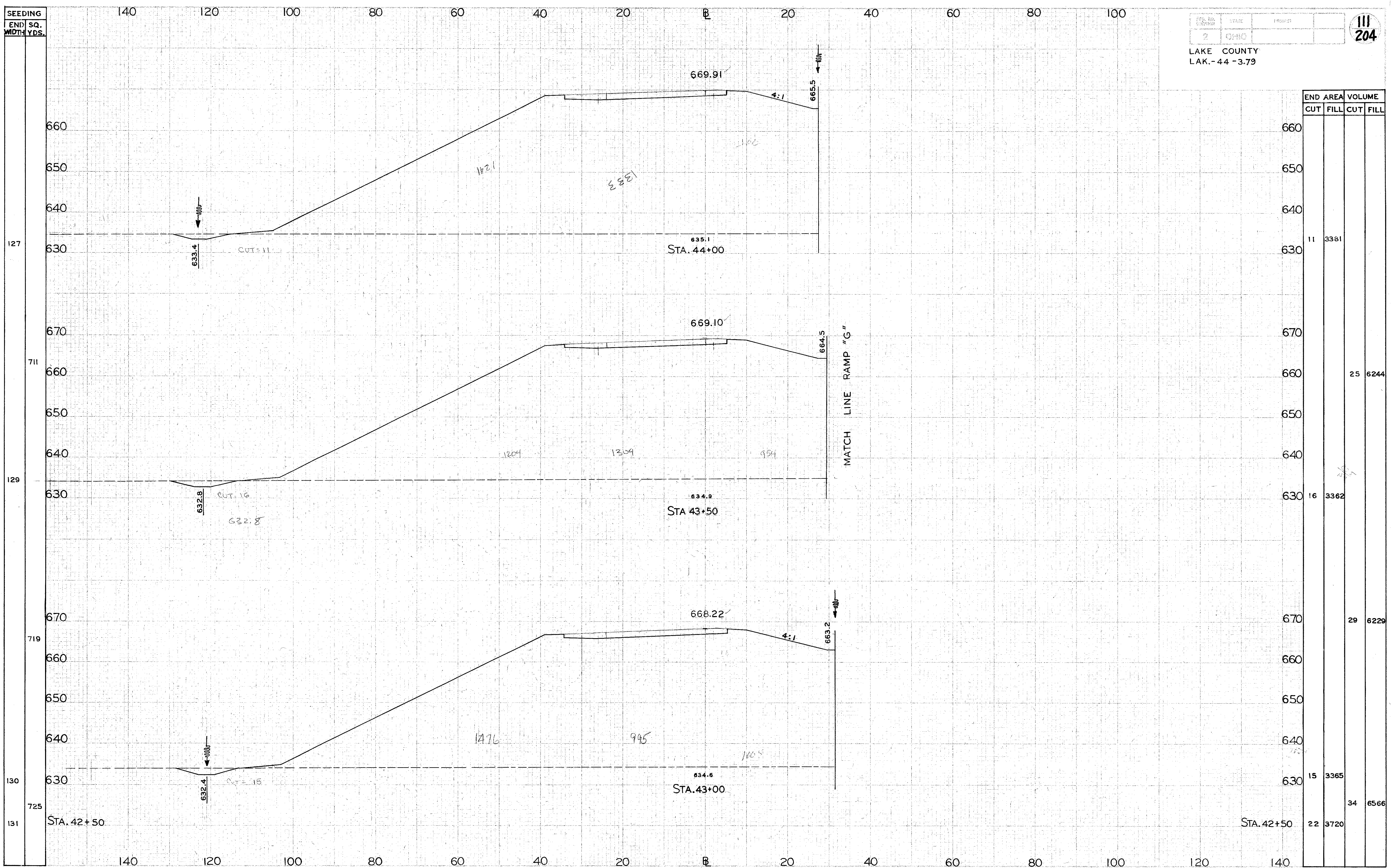
RAMP "E" STA. 43+00 TO STA. 44+00
