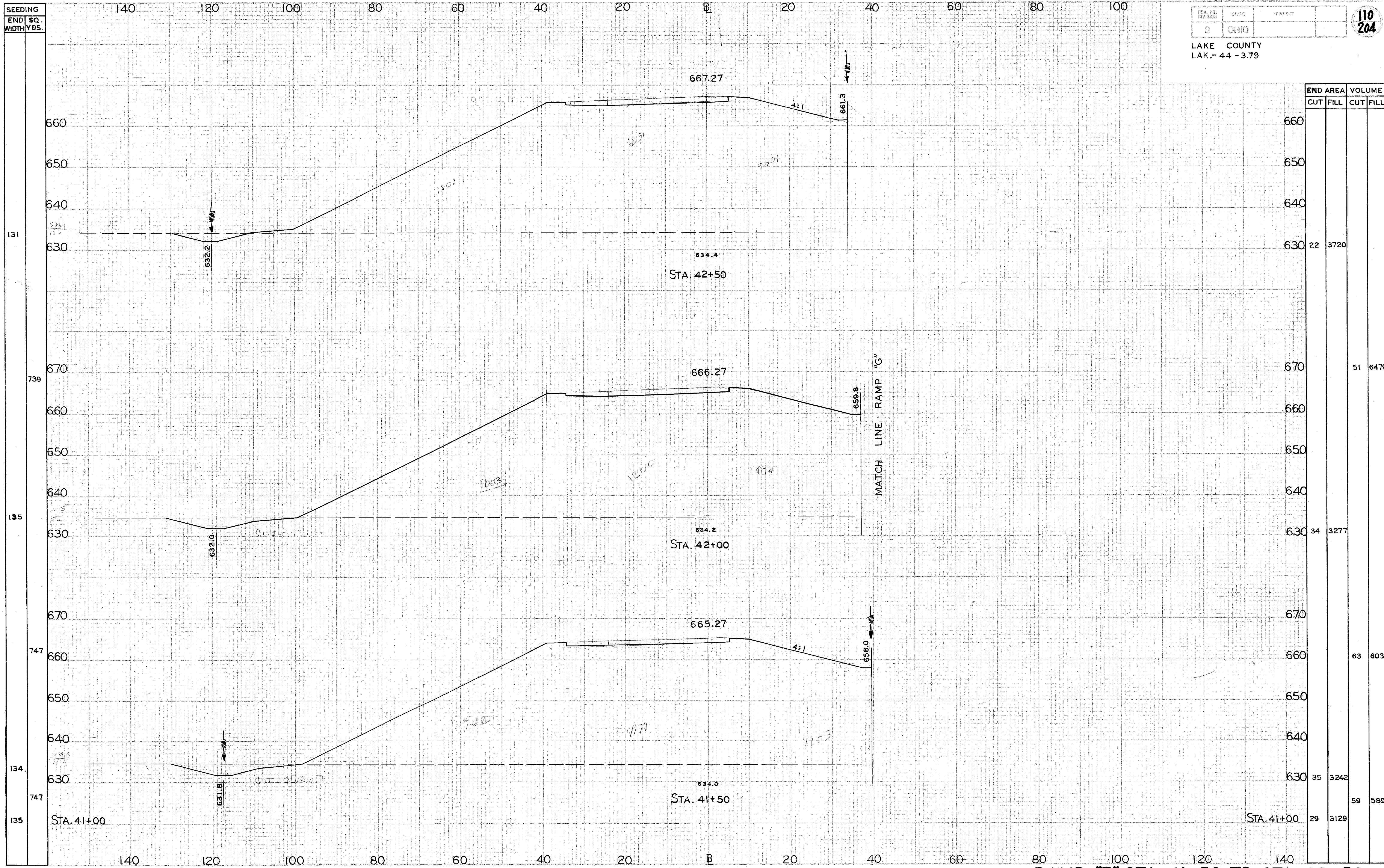
RAMP "E" STA. 41+50 TO STA. 42+50
