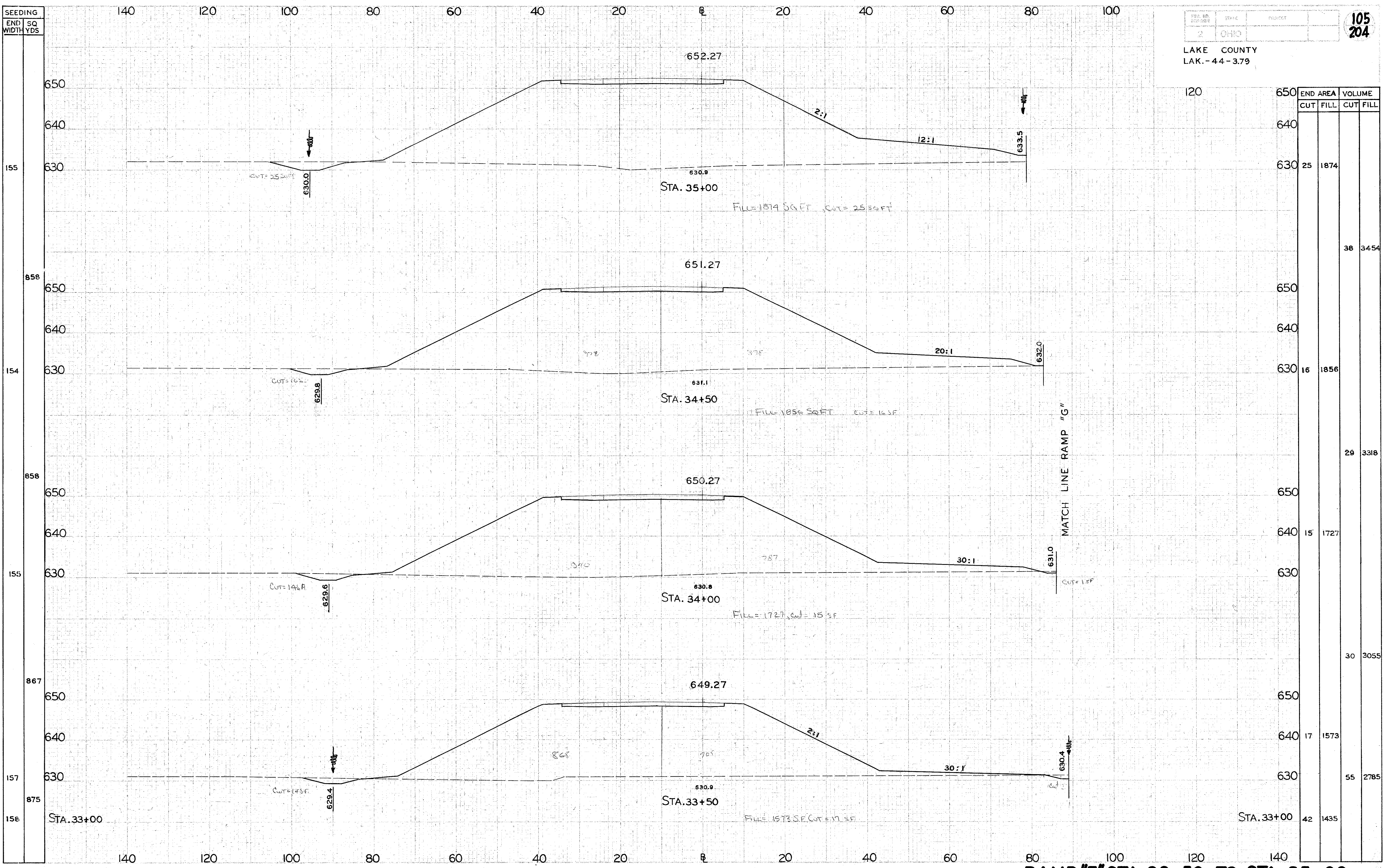
RAMP "E" STA. 33+50 TO STA. 35+00
