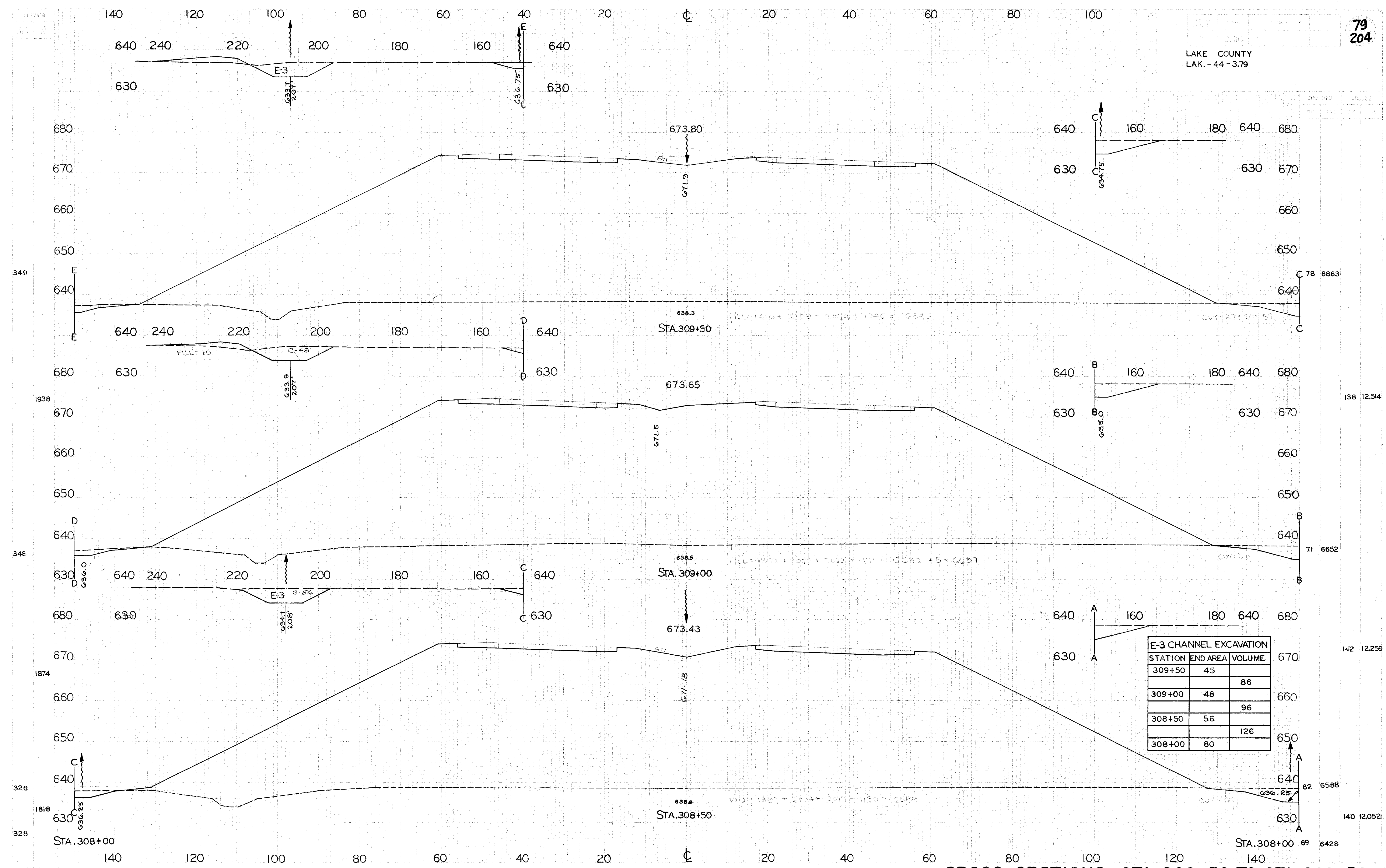
CROSS SECTIONS STA. 308+50 TO STA. 309+50
