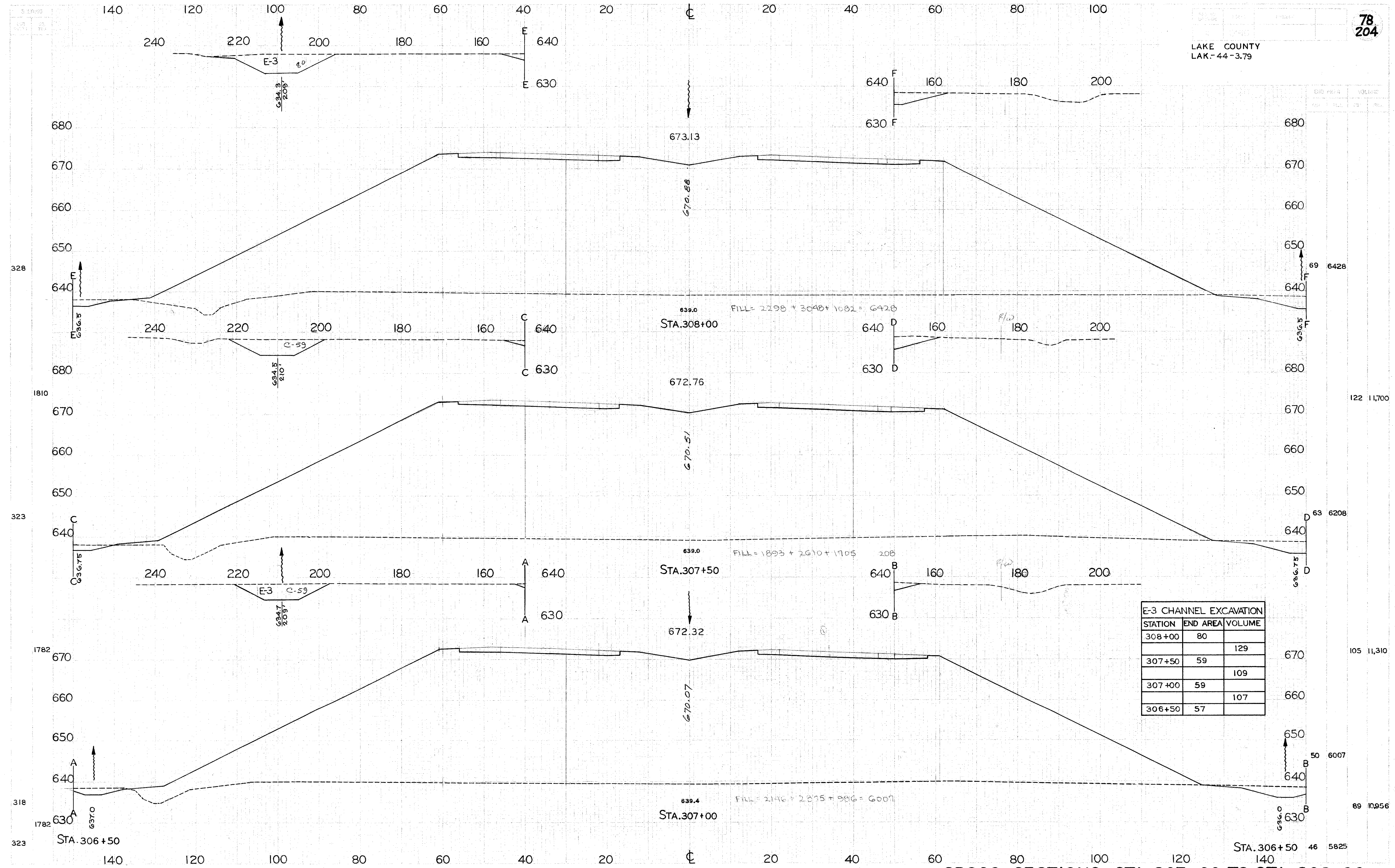
CROSS SECTIONS STA. 307+00 TO STA. 308+00
