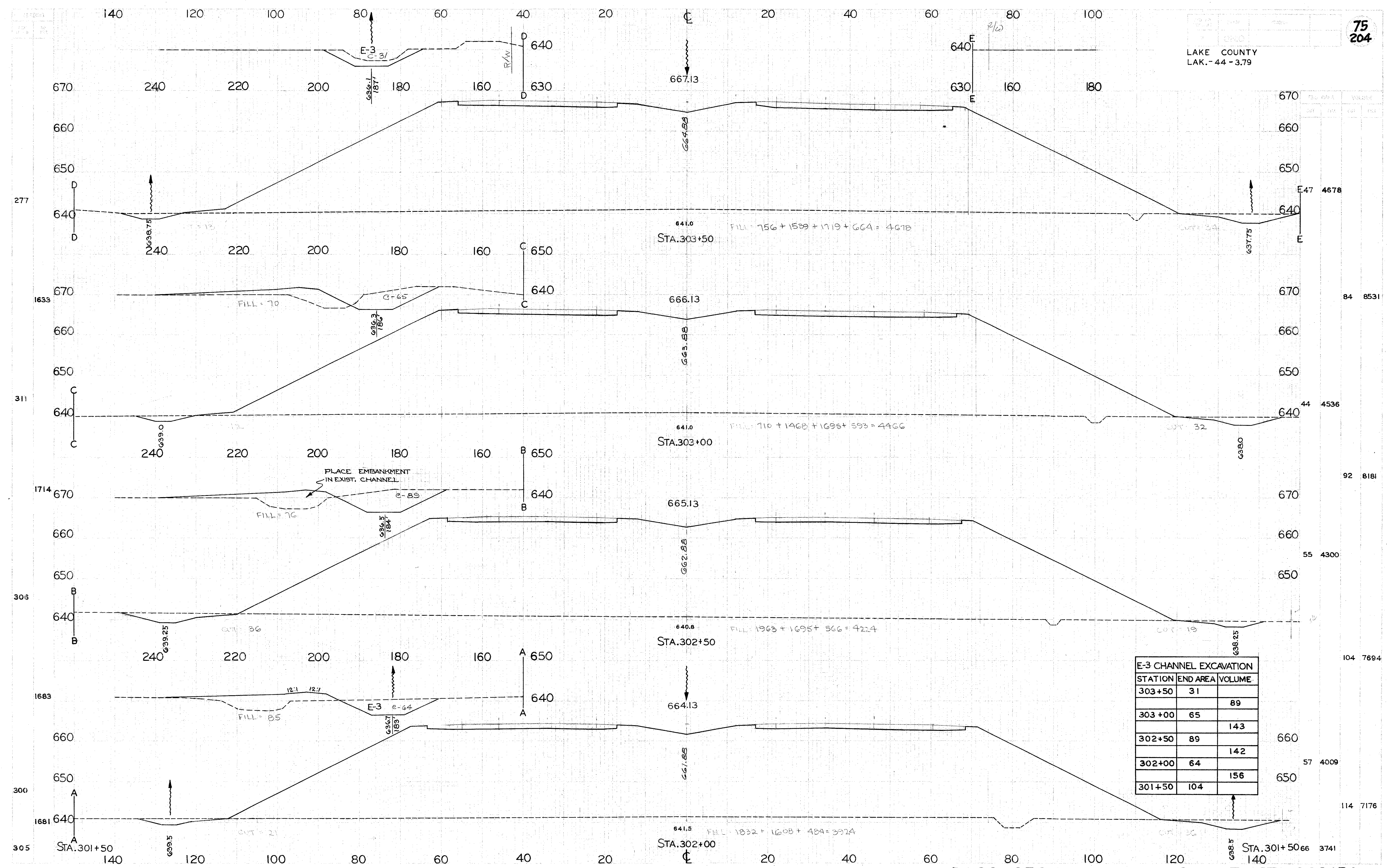
CROSS SECTIONS STA. 302+00 TO STA. 303+50
