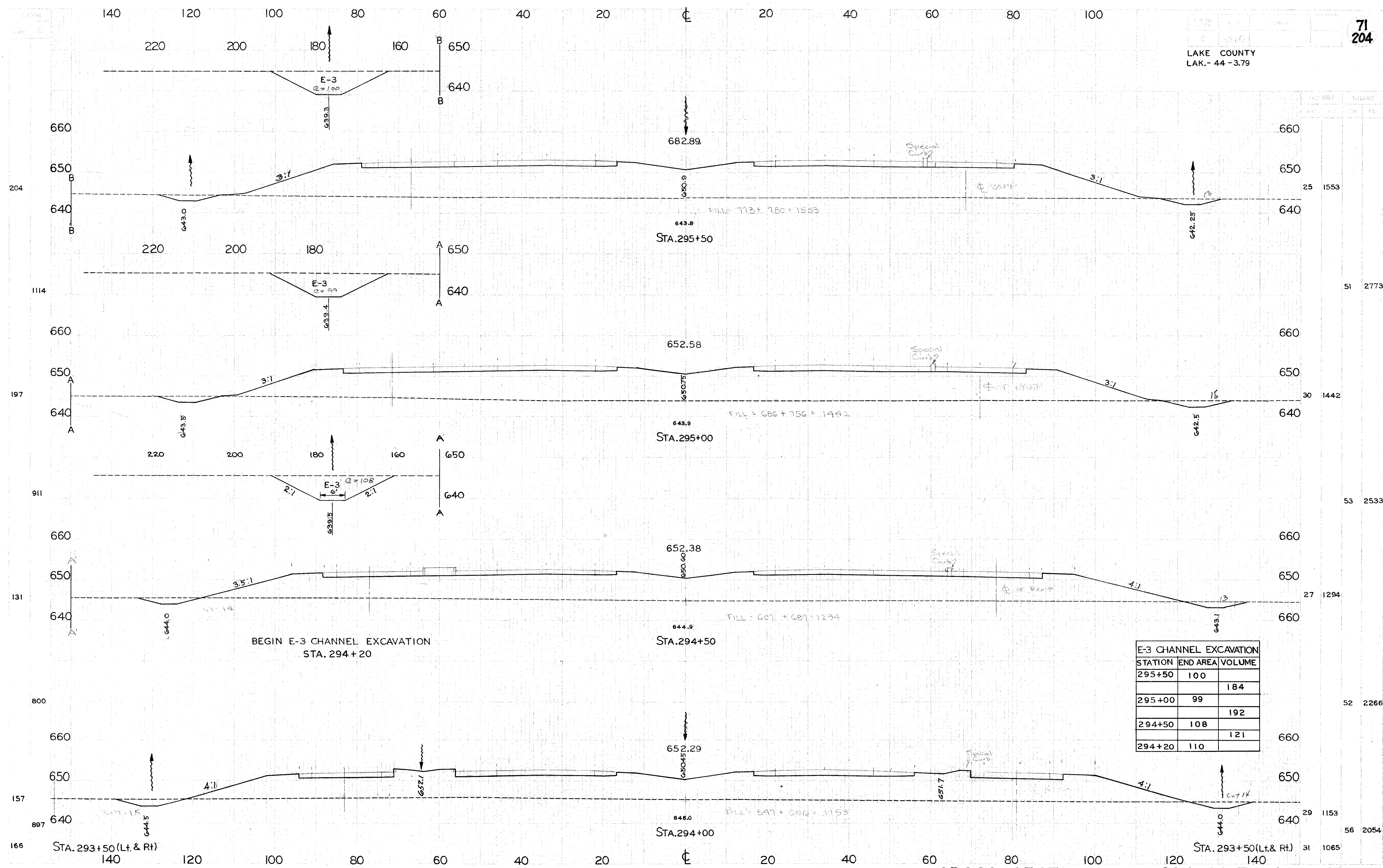
CROSS SECTIONS STA. 294+00 TO STA. 295+50
