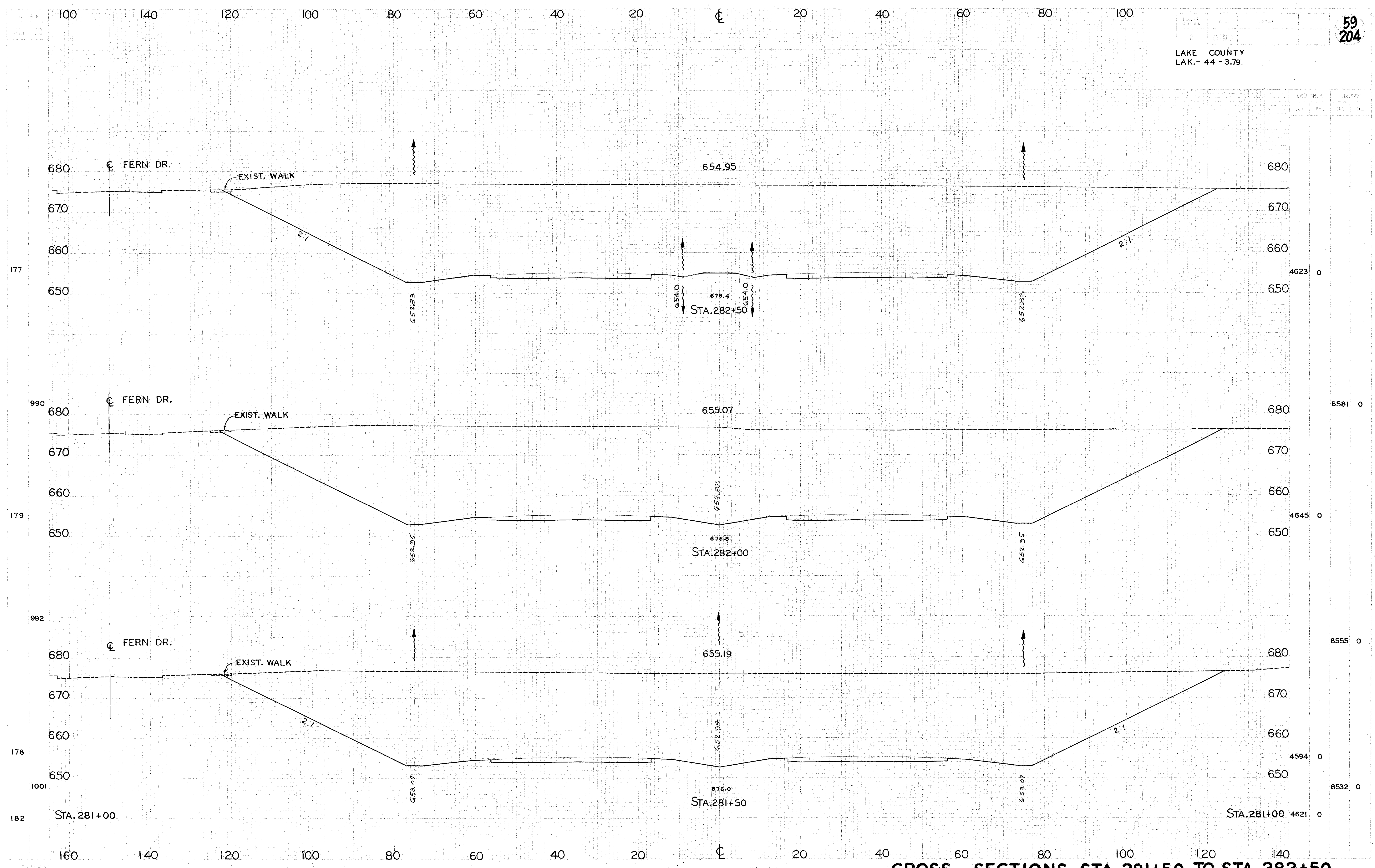
CROSS SECTIONS STA. 281+50 TO STA. 282+50
