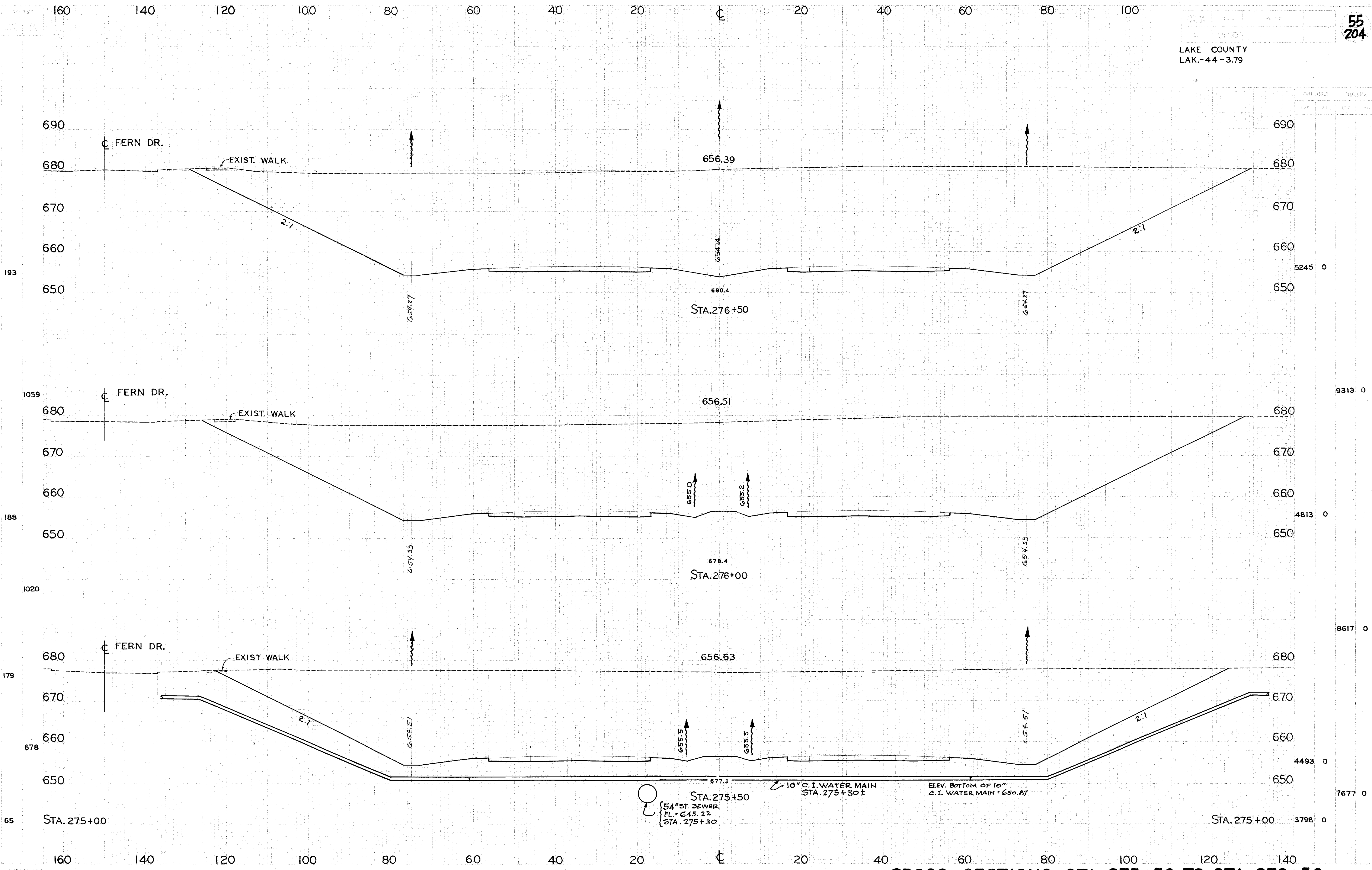
CROSS SECTIONS STA. 275+50 TO STA. 276+50
