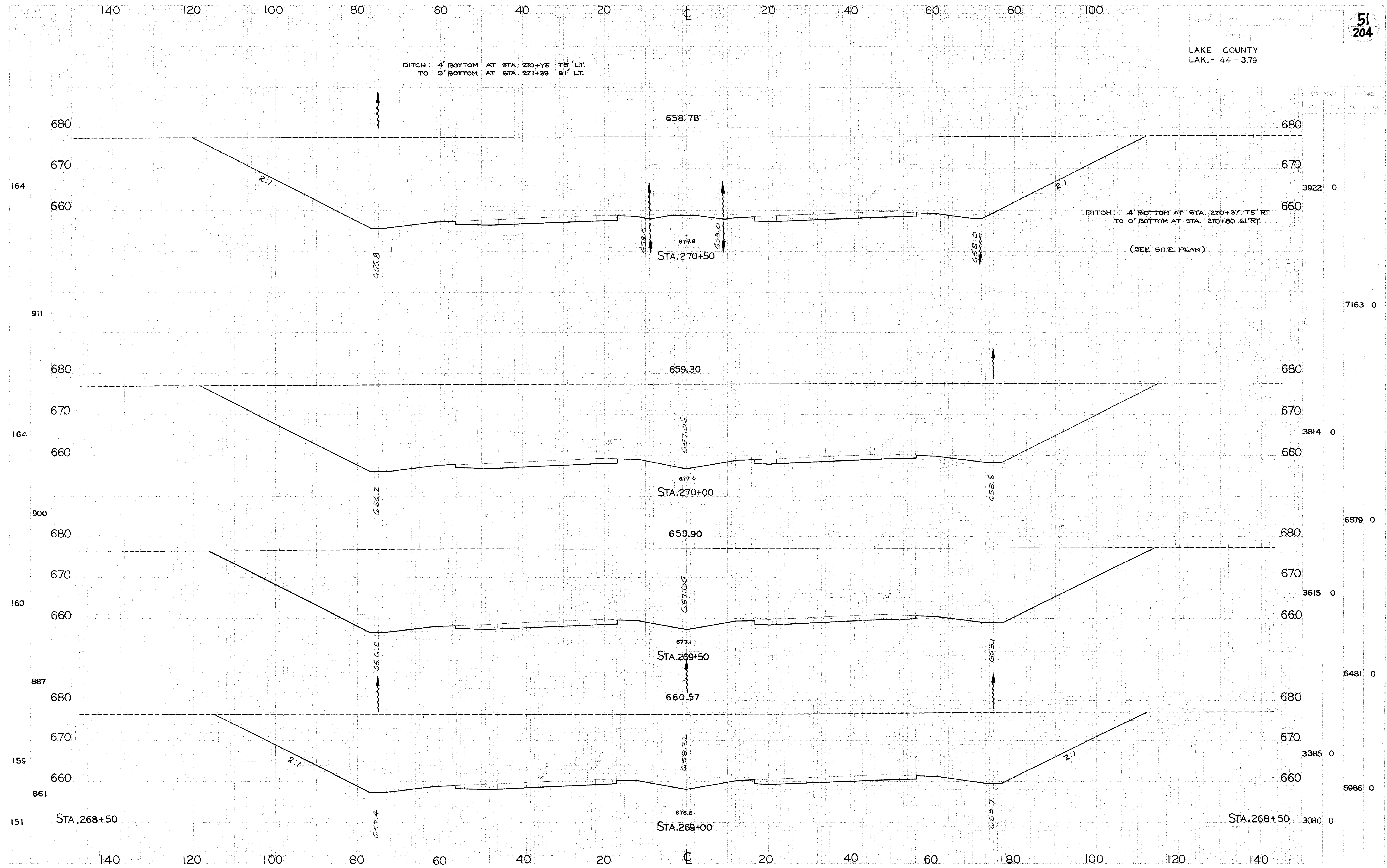
CROSS SECTIONS STA. 269+00 TO STA. 270+50
