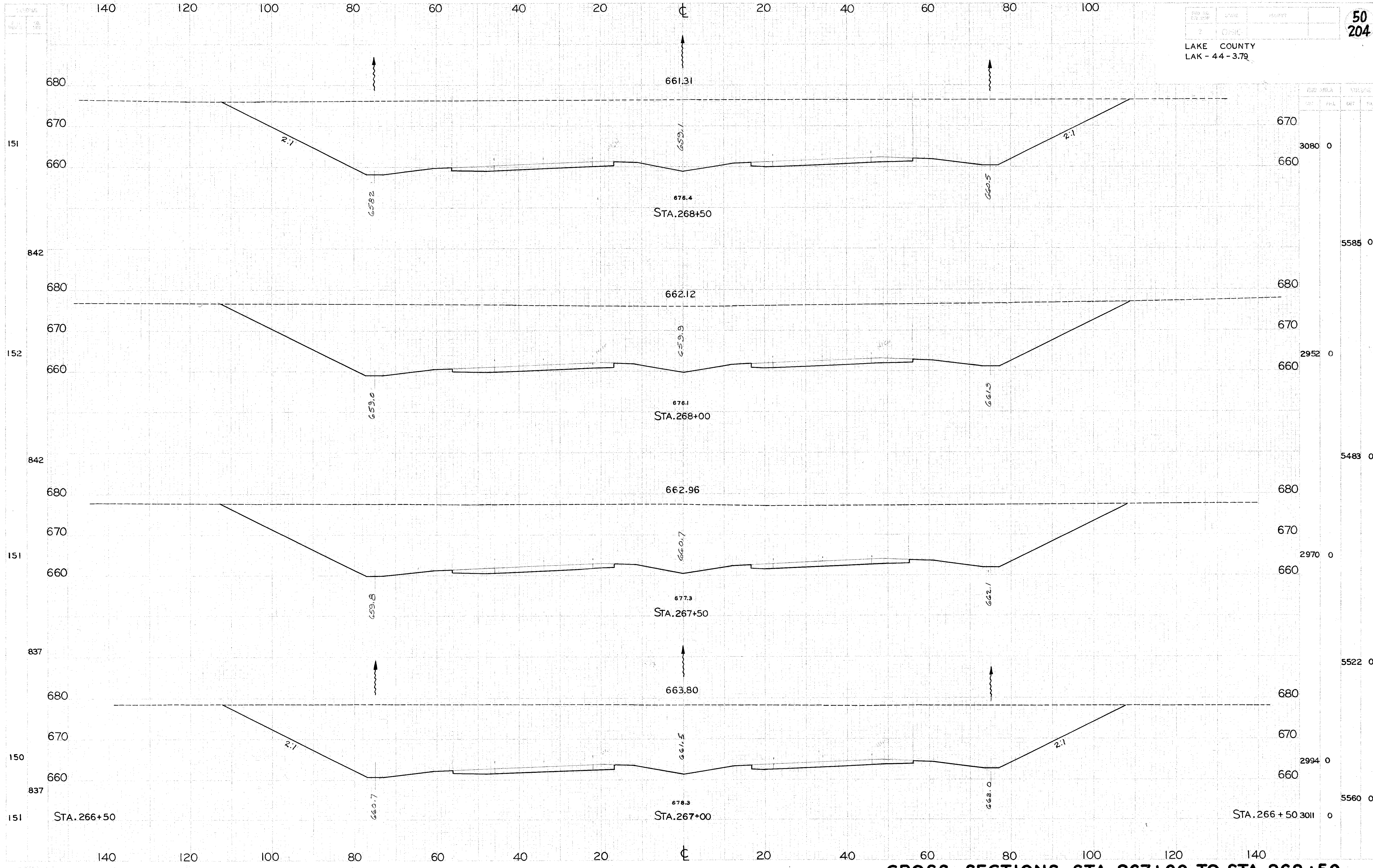
CROSS SECTIONS STA. 267+00 TO STA. 268+50
