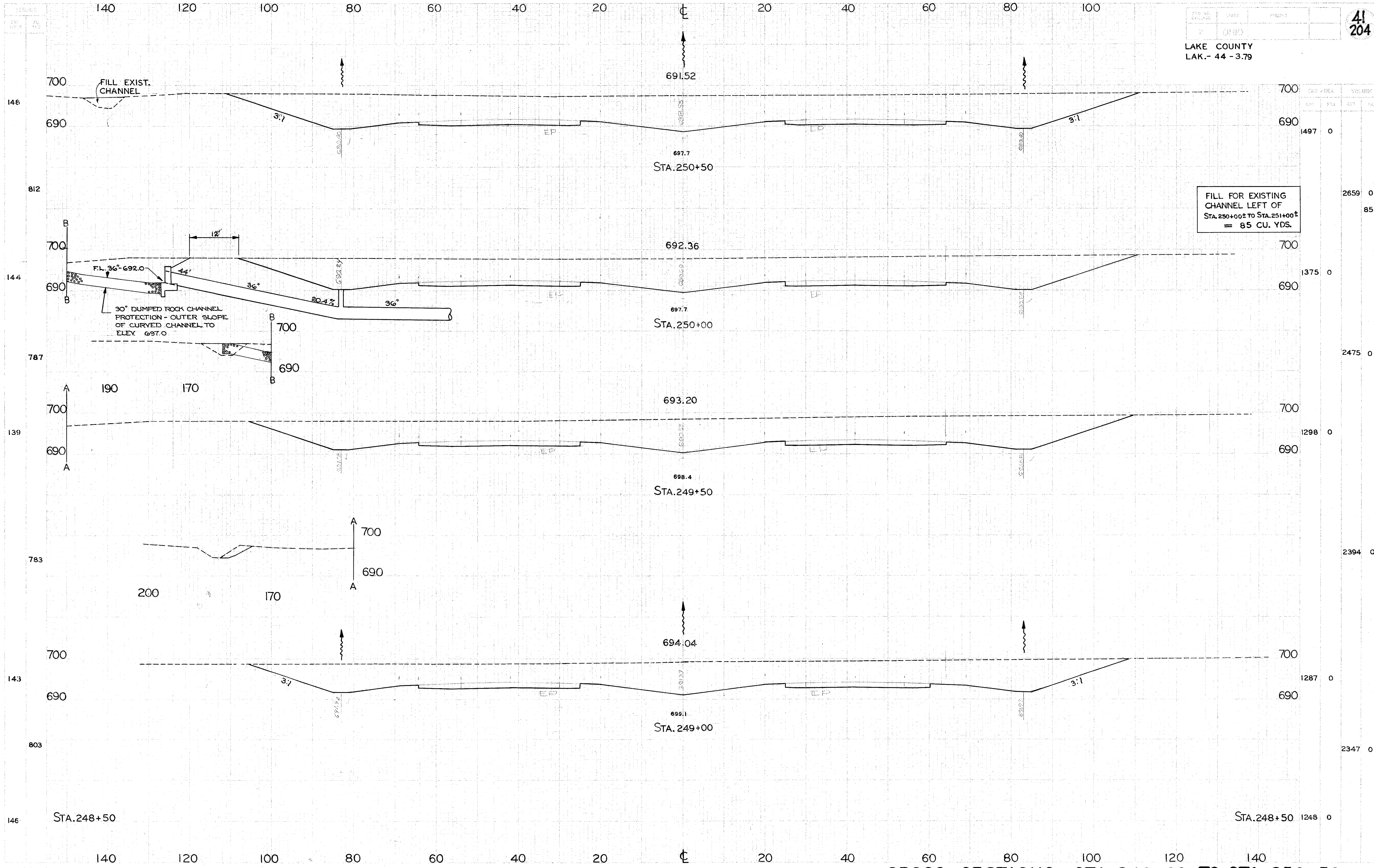
CROSS SECTIONS STA. 249+00 TO STA. 250+50
