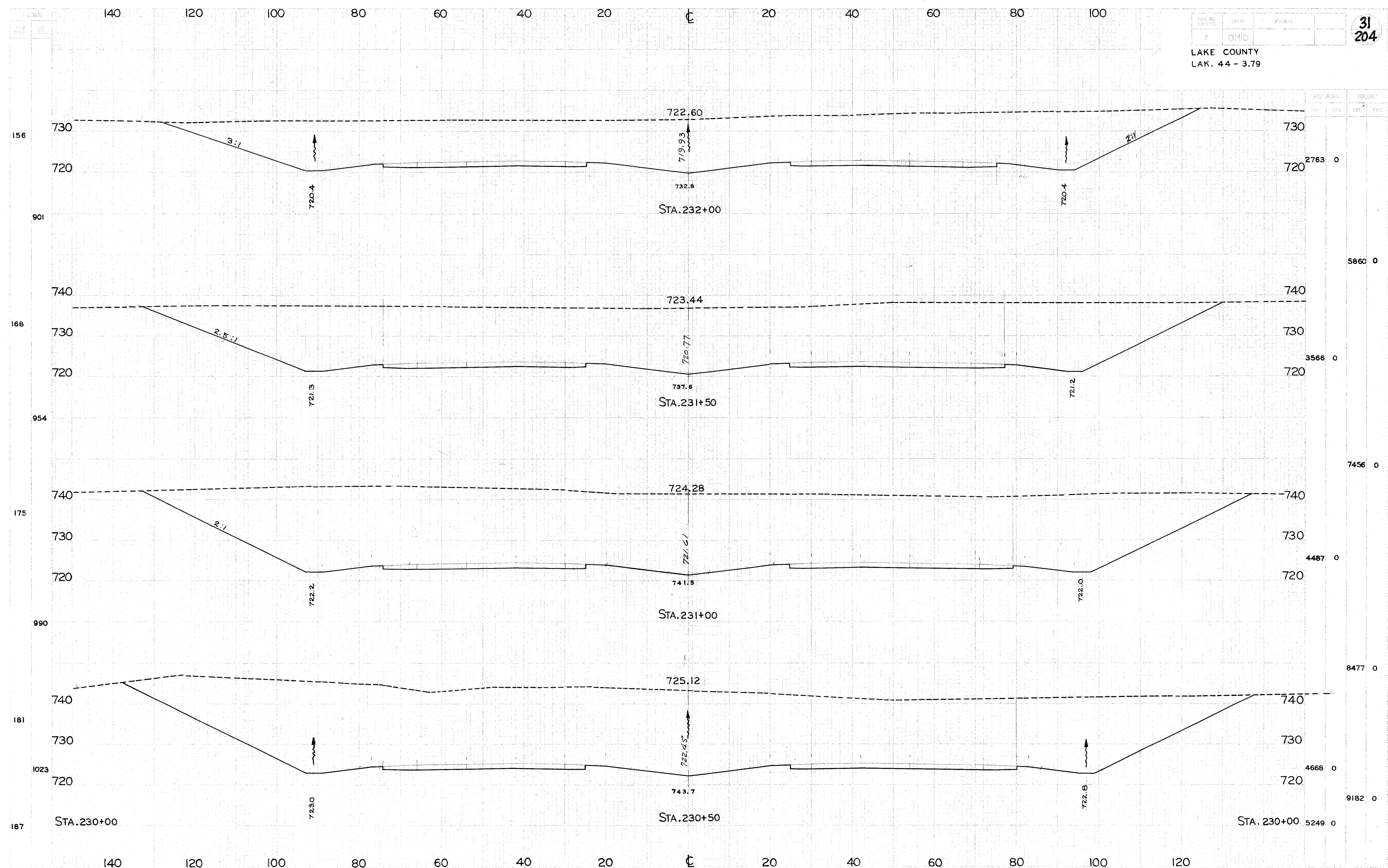
CROSS SECTIONS STA. 230+50 TO STA. 232+00
