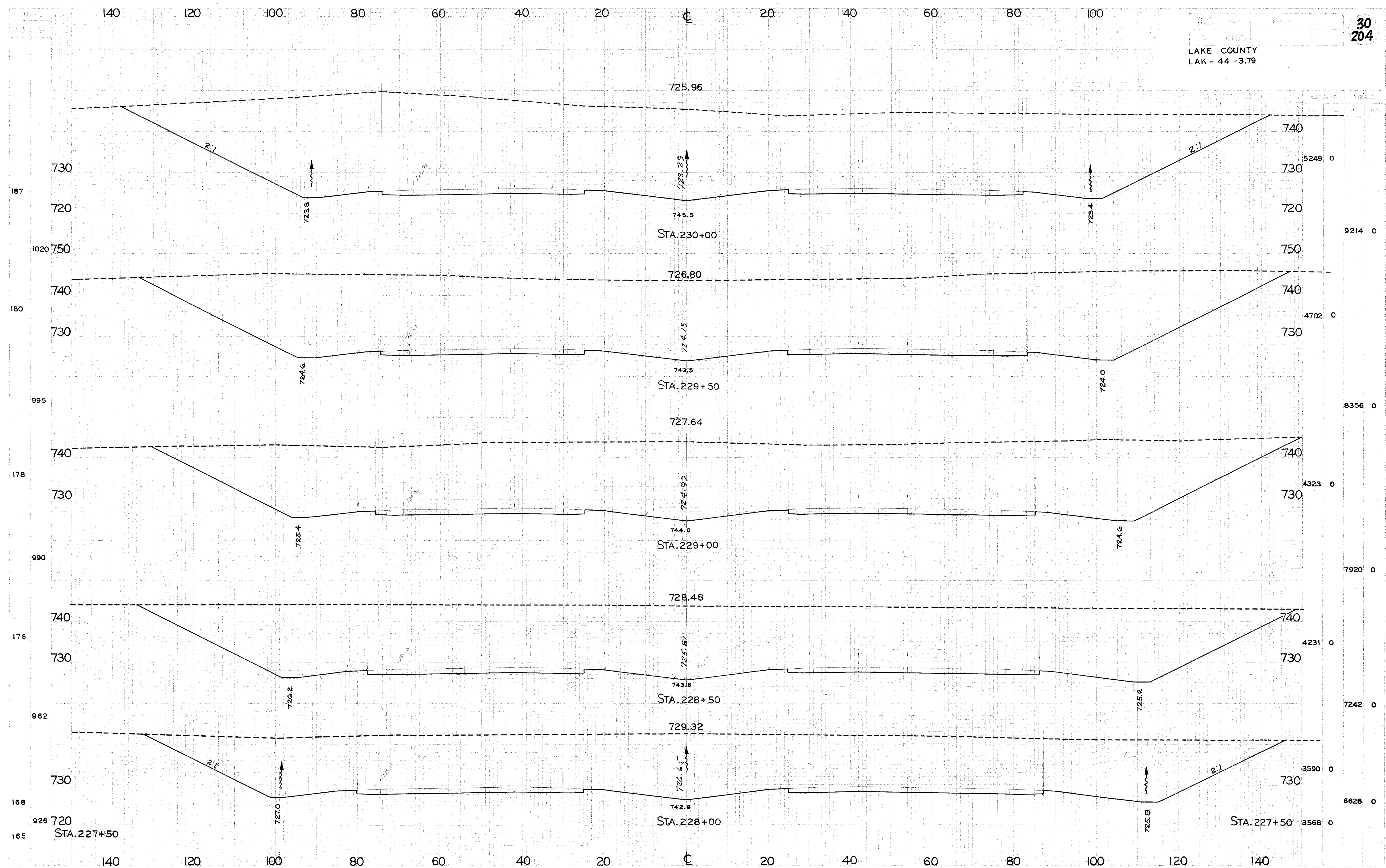
CROSS SECTIONS STA. 228+00 TO STA. 230+00
