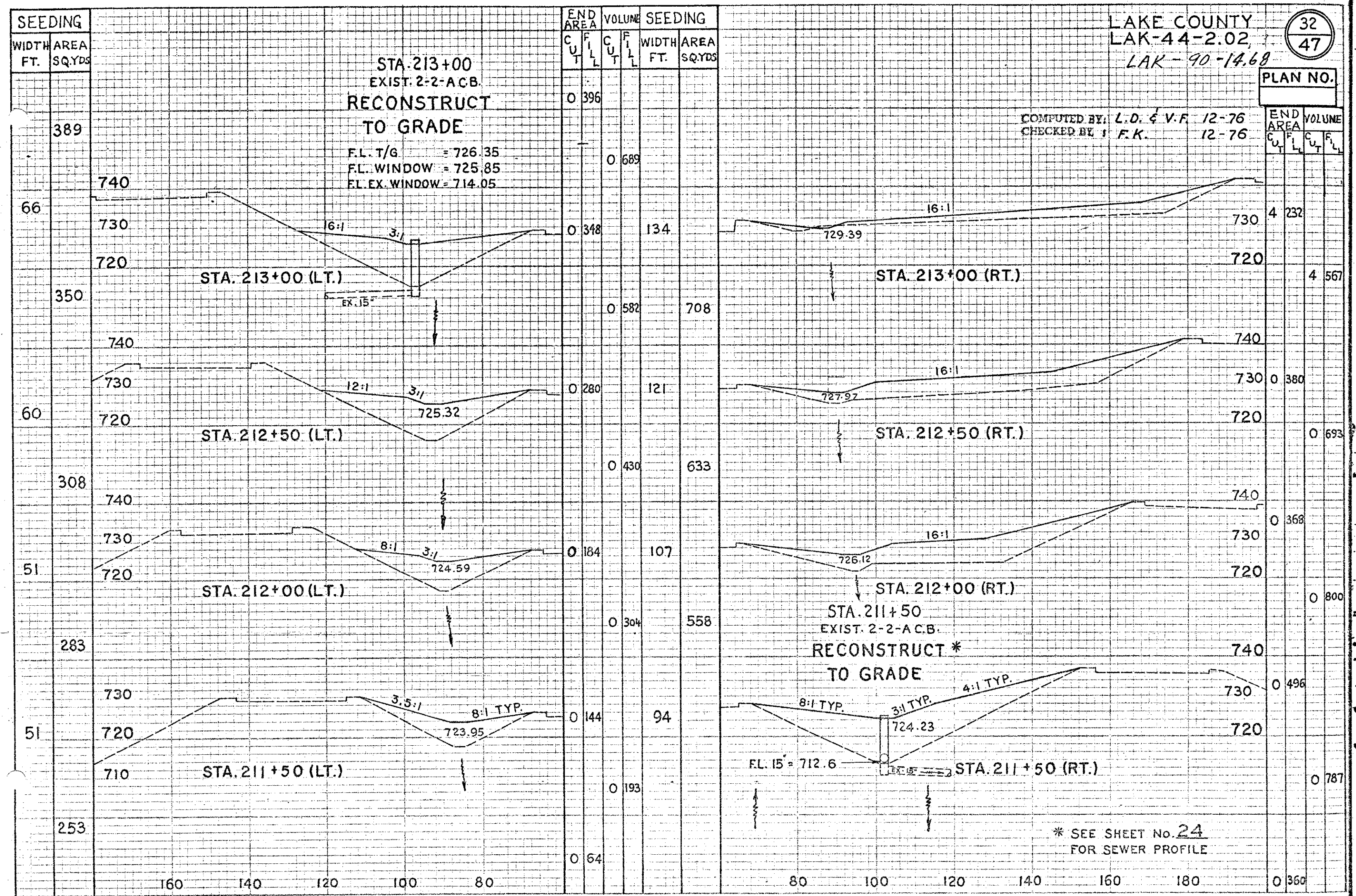
X-SECTIONS STA. 211+50 to STA. 213+00
