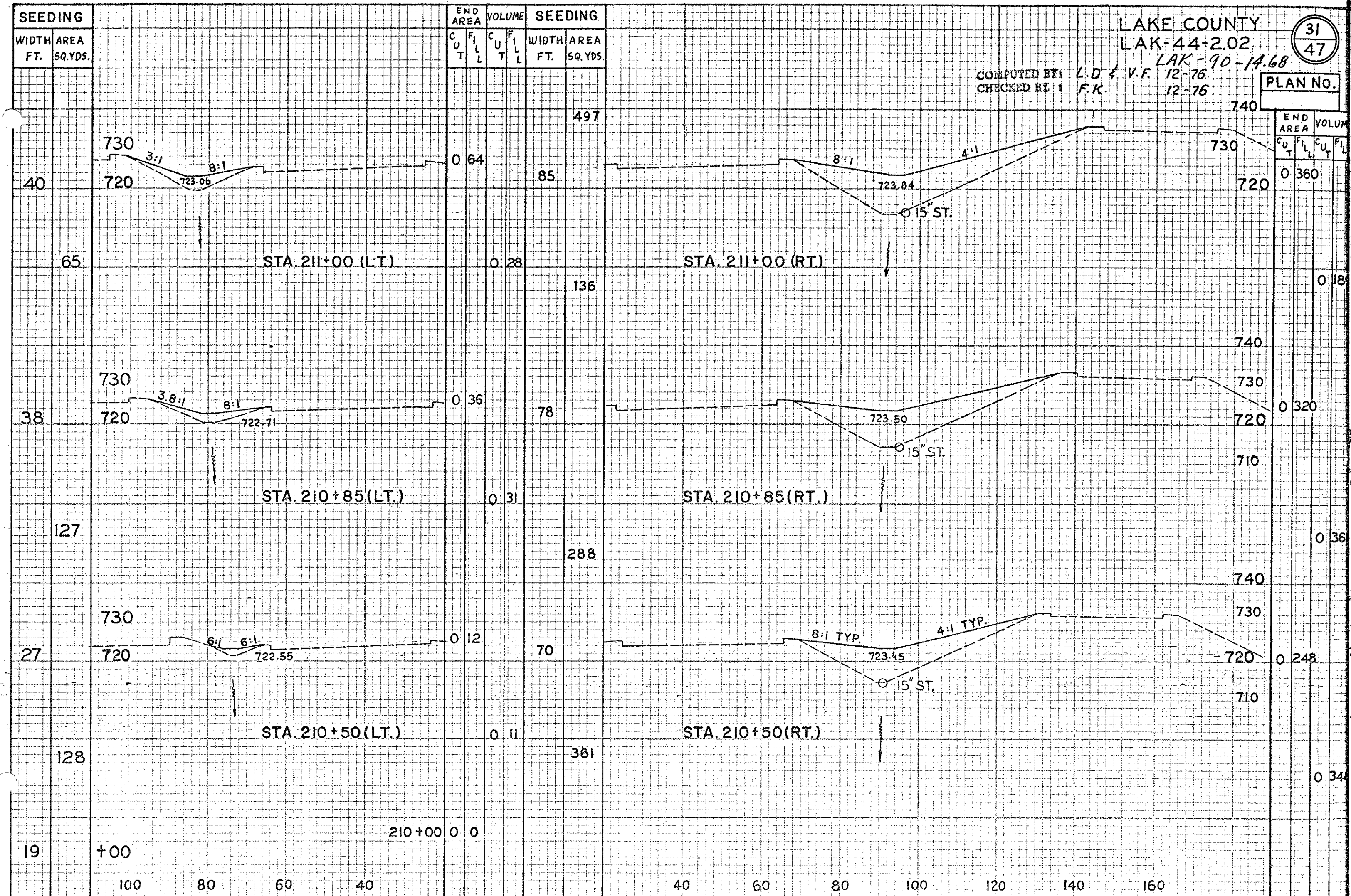
X-SECTIONS STA. 210+50 to STA. 211+00
